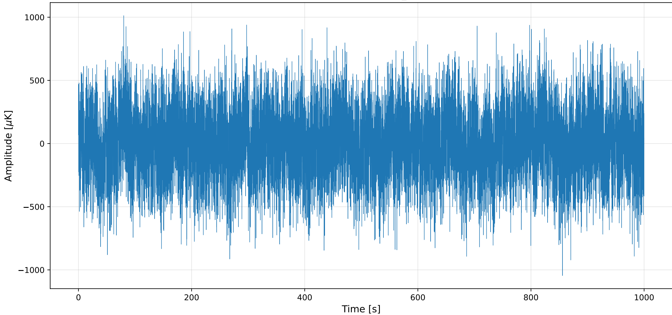
TOD: Mock Detector (add_lbsNoise)
