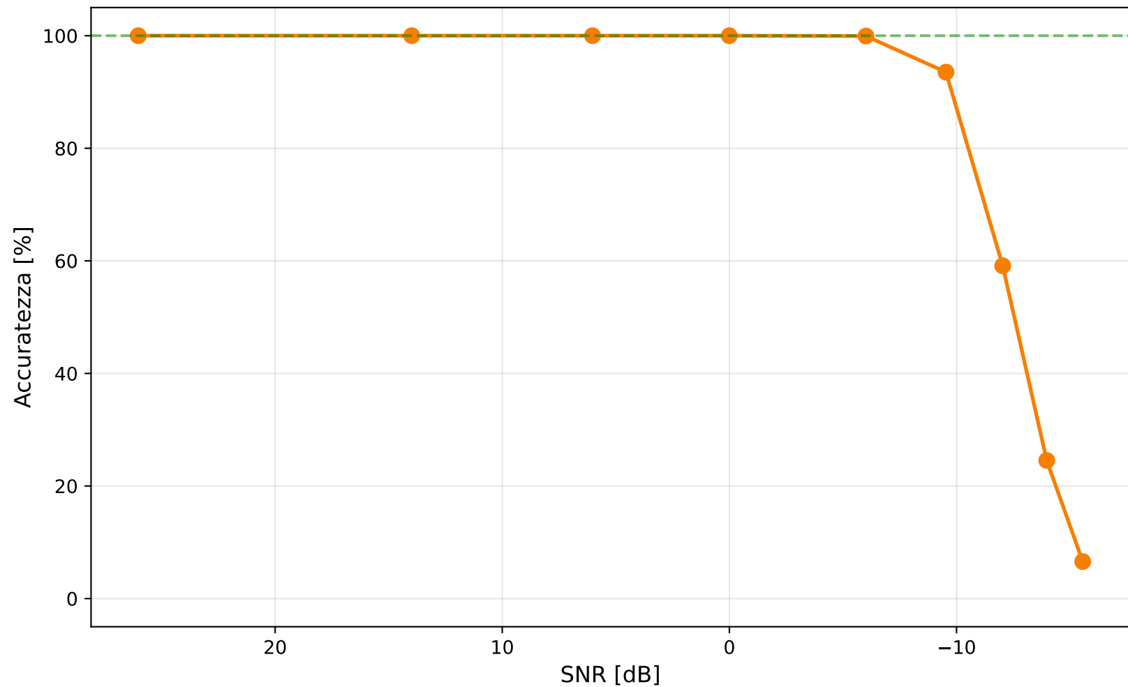
Accuratezza di riconoscimento DTMF in funzione del SNR
