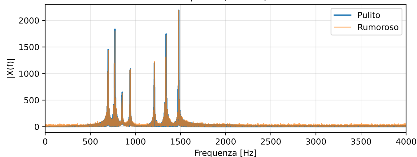
Spettro ( \sigma = 0.5 )
