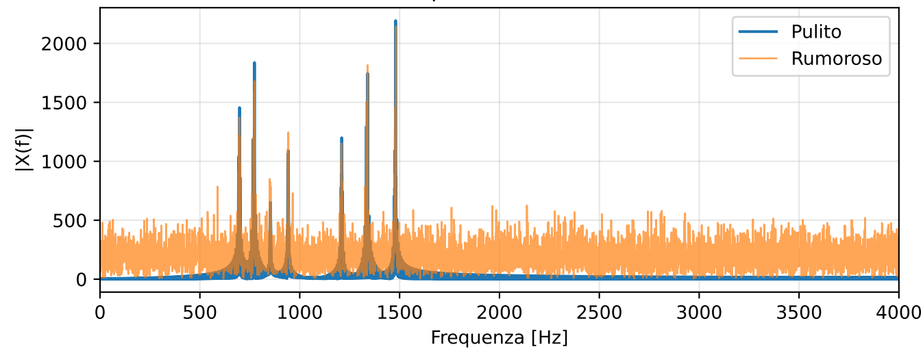
Spettro ( \sigma = 2 )
