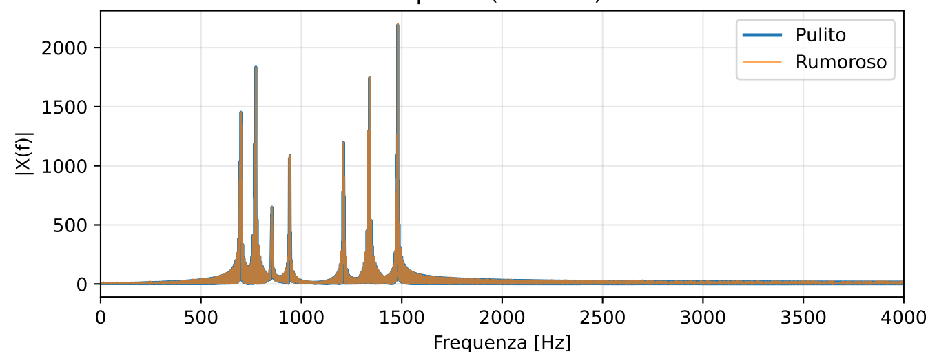
Spettro ( \sigma = 0.2 )
