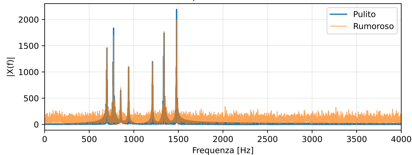
Spettro ( \sigma = 2 )
