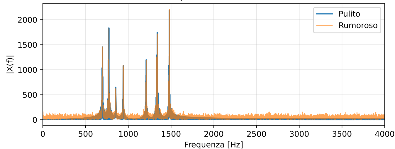
Spettro ( \sigma = 1 )
