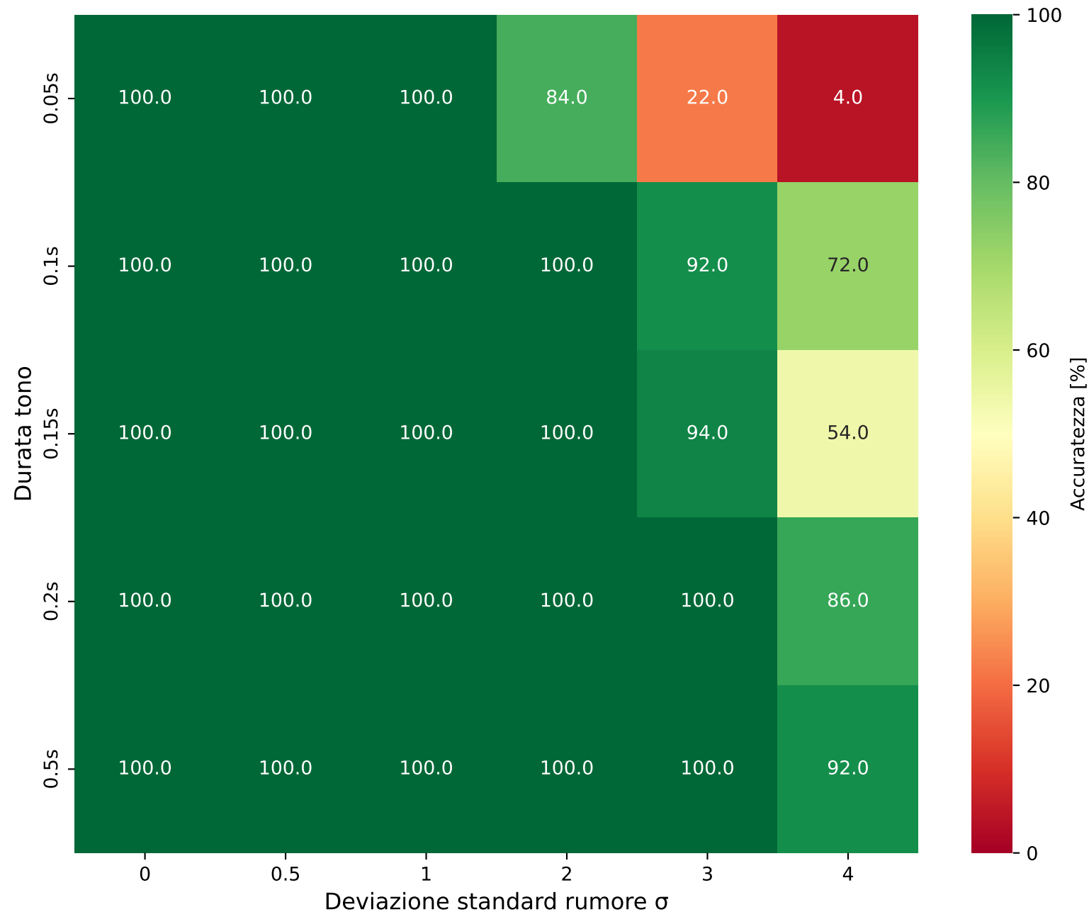
Accuratezza riconoscimento DTMF vs Durata e Livello di Rumore
