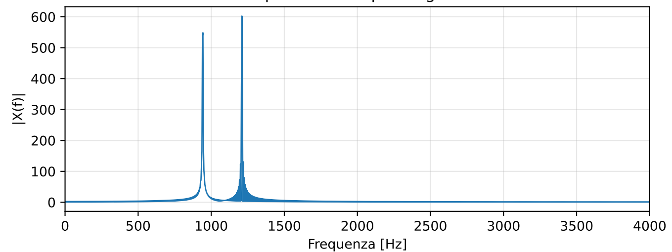
Spettro - Zero-padding 4x
