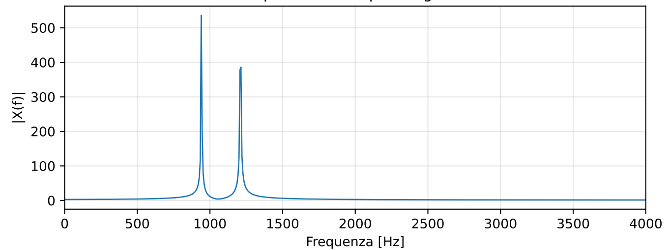
Spettro - Zero-padding 2x
