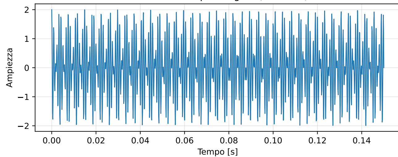
Tono '*' - Zero-padding 2x (M=2400)
