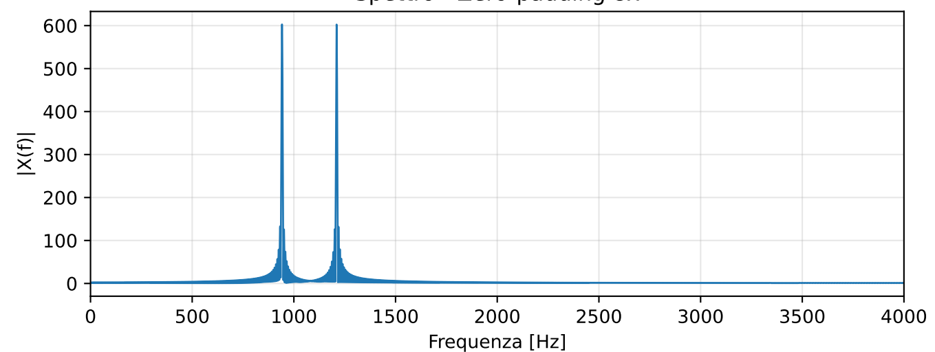
Spettro - Zero-padding 8x
