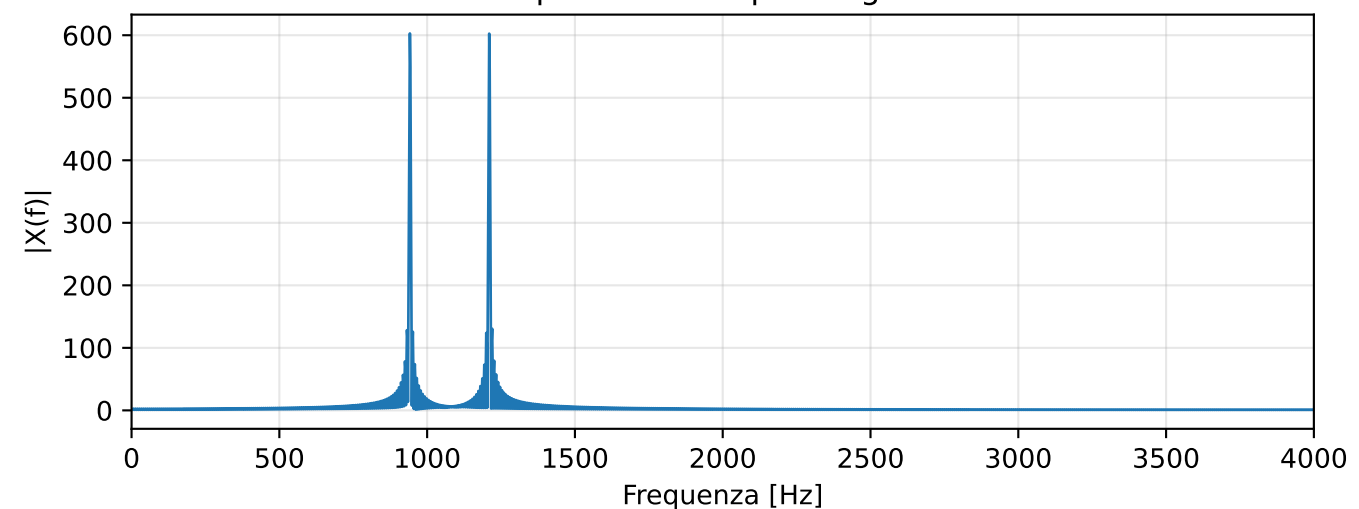
Spettro - Zero-padding 8x
