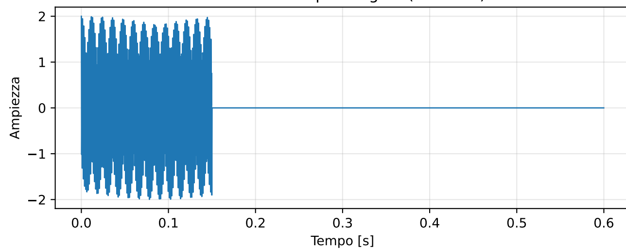
Tono '3' - Zero-padding 8x (M=9600)
