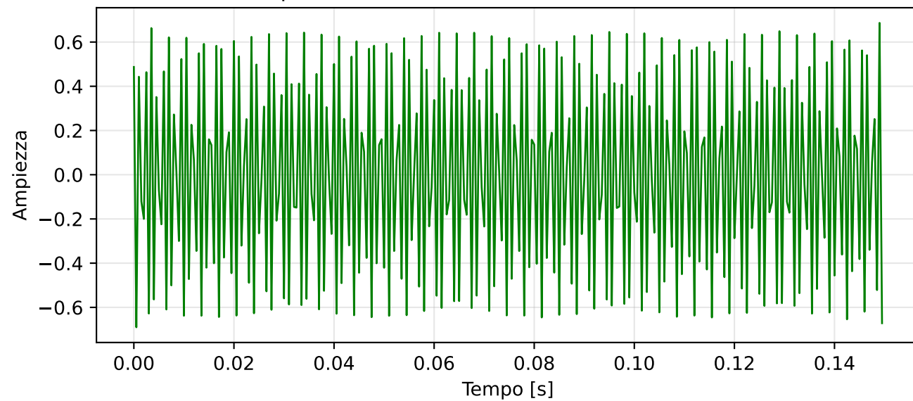
Ricampionamento con filtro anti-alias - F_s = 2000 Hz
