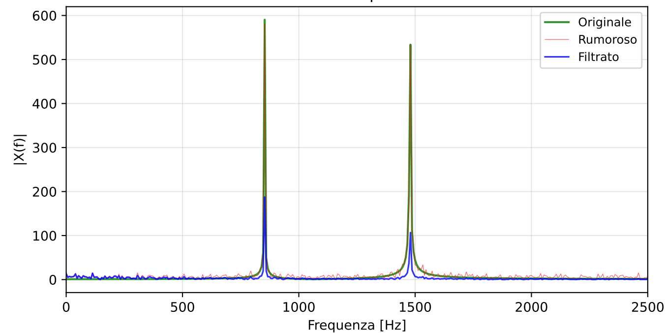
Dominio della frequenza - \sigma=0.5
