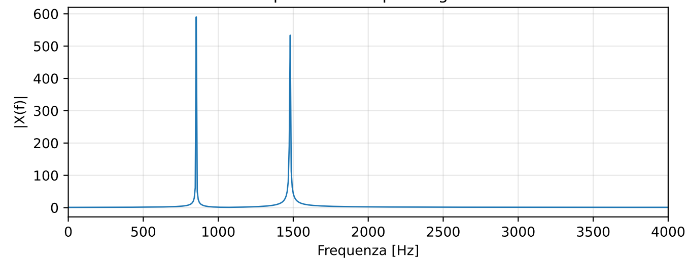
Spettro - Zero-padding 2x
