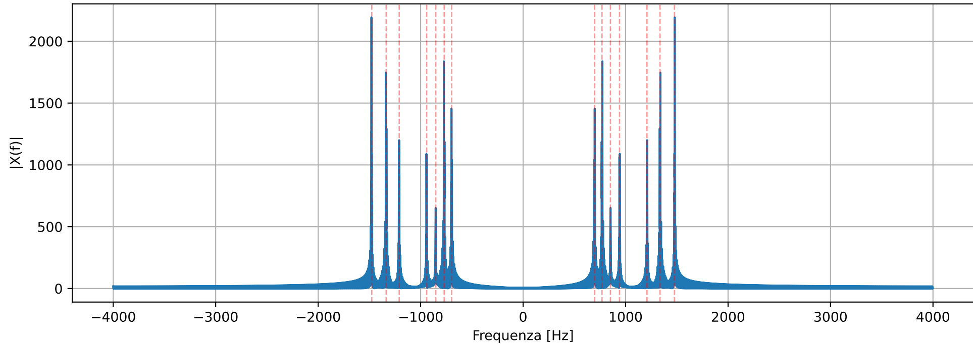
Spettro DTMF
