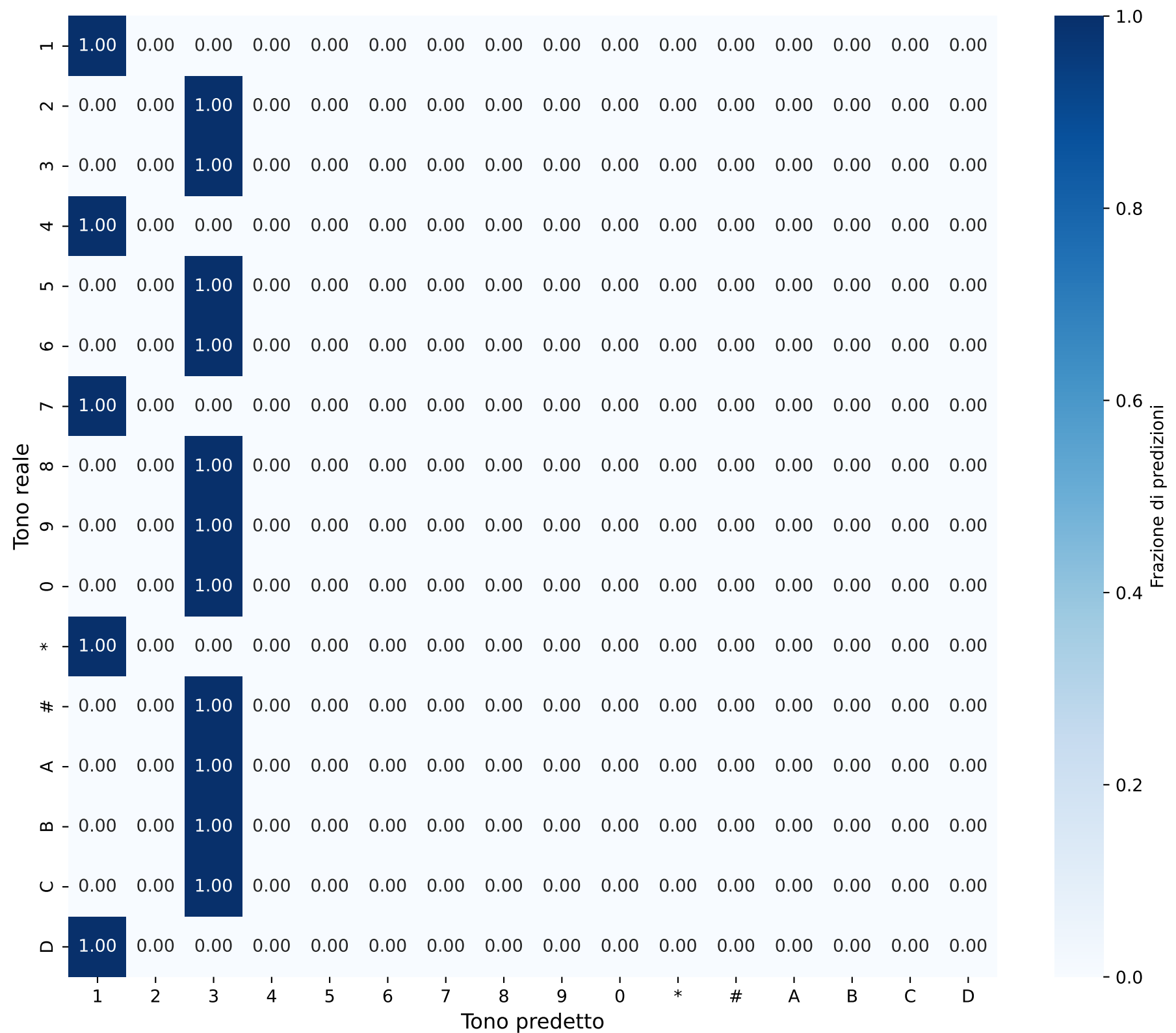
Matrice di Confusione - Sequenze Durata: 0.0026s
