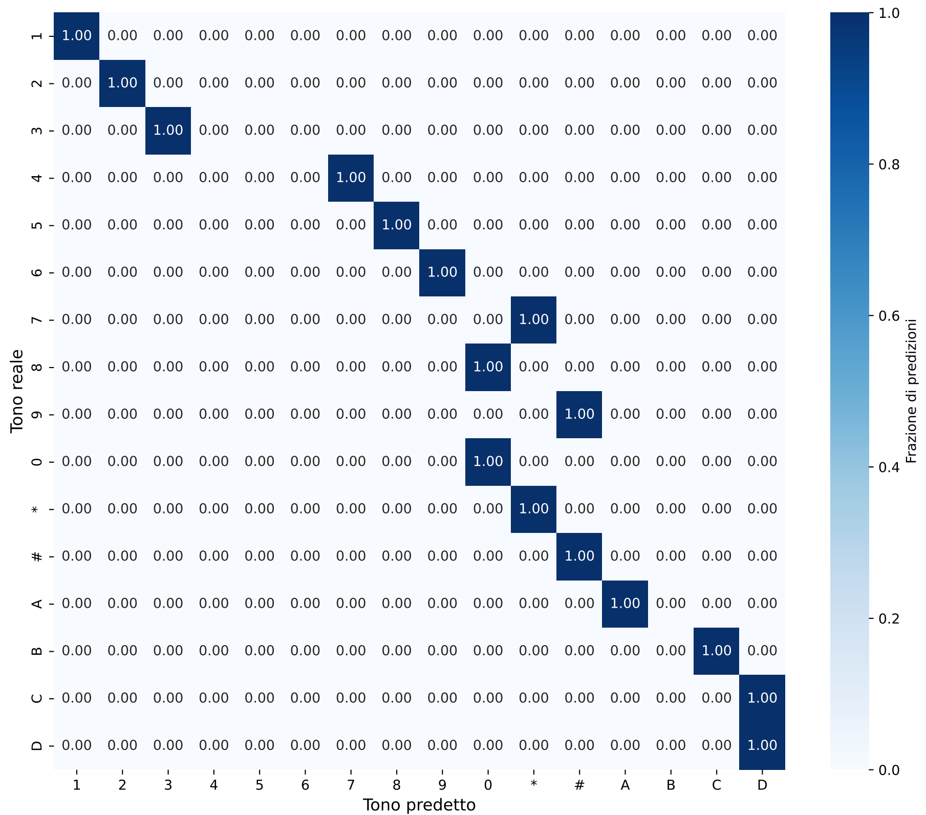
Matrice di Confusione - Singoli Toni Durata: 0.0111s
