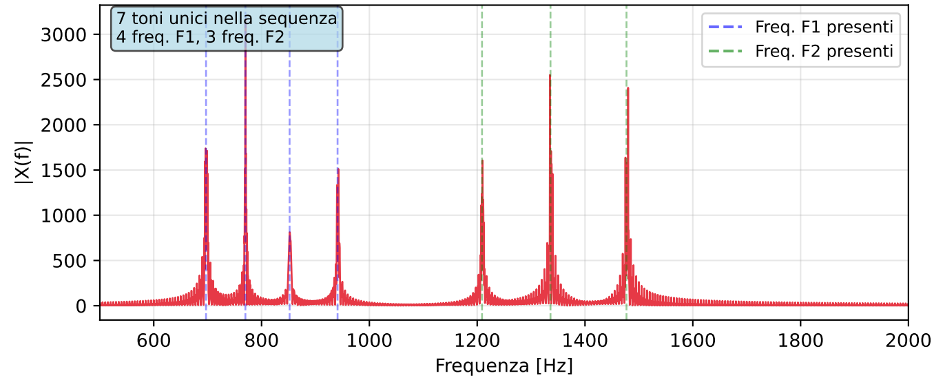
Spettro della sequenza - Risoluzione \Delta f = 5.0 Hz
