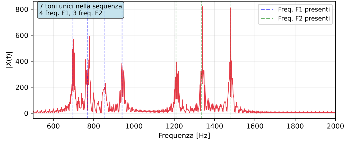
Spettro della sequenza - Risoluzione \Delta f = 20.0 Hz
