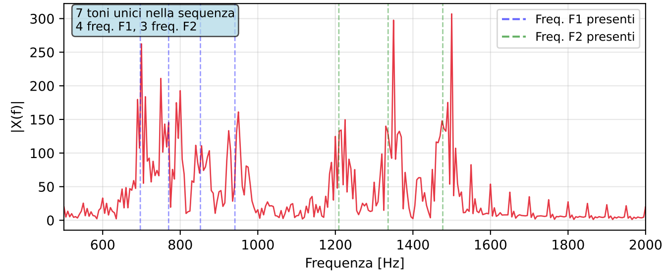
Spettro della sequenza - Risoluzione \Delta f = 50.0 Hz
