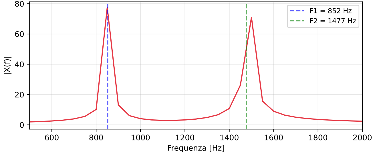
Spettro - Risoluzione \Delta f = 50.0 Hz
