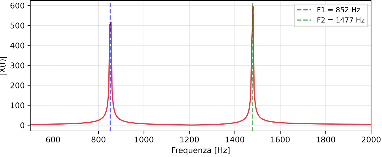
Spettro - Risoluzione \Delta f = 5.0 Hz
