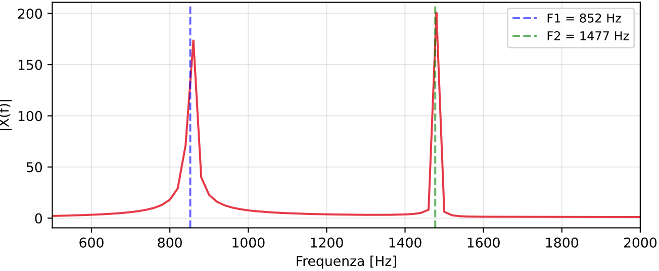
Spettro - Risoluzione \Delta f = 20.0 Hz
