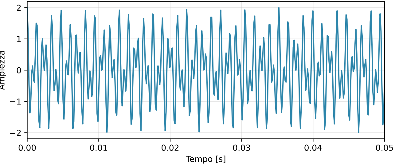
Tono '9' - Durata: 0.1s (800 campioni)
