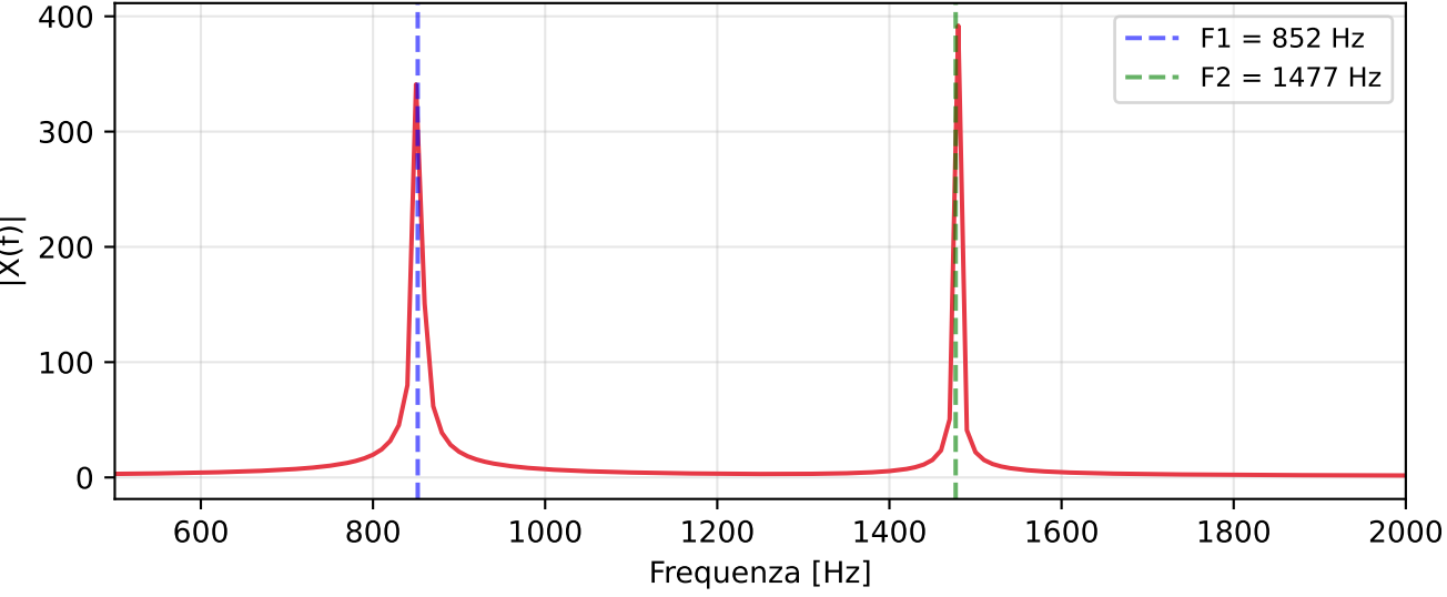
Spettro - Risoluzione \Delta f = 10.0 Hz
