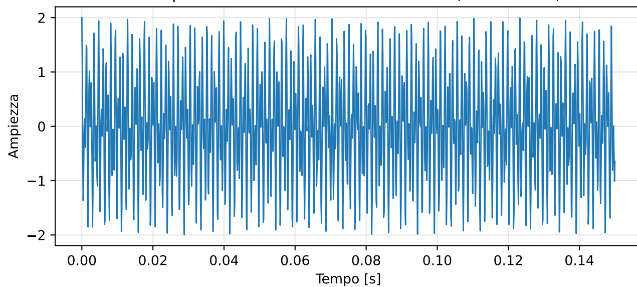
Campionamento diretto - F_s = 2000 Hz (Aliasing)
