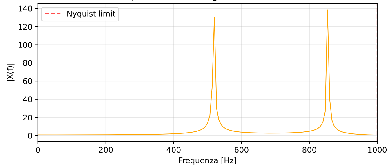
Spettro filtrato (no aliasing) - F_s = 2000 Hz
