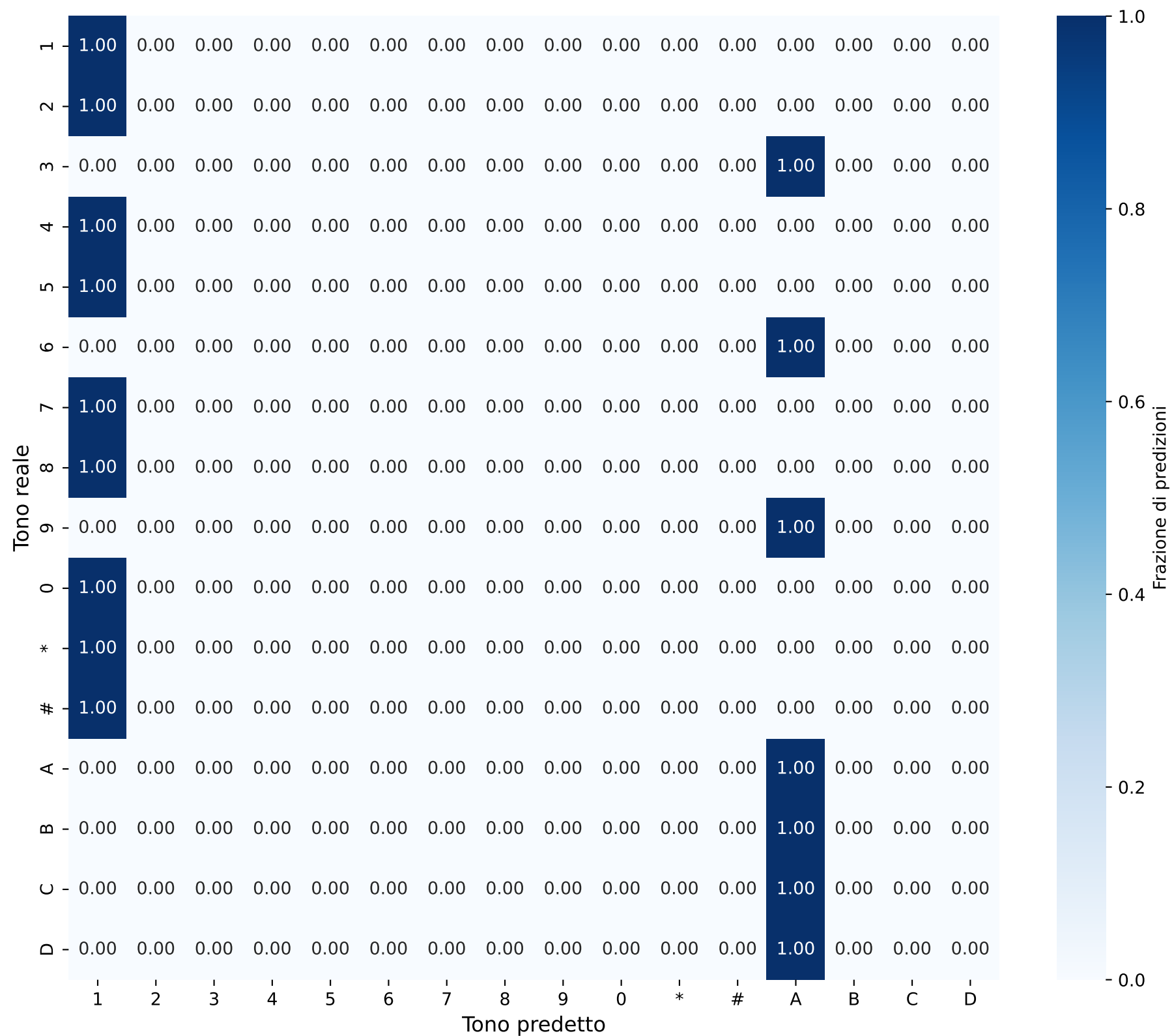
Matrice di Confusione - Sequenze Durata: 0.001s
