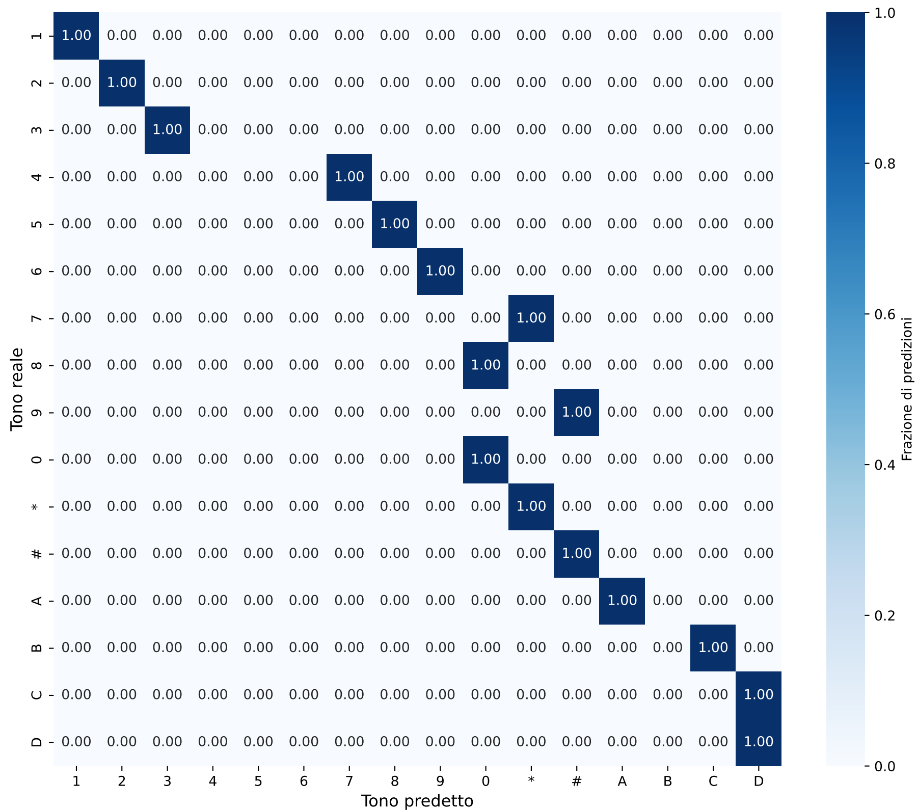
Matrice di Confusione - Sequenze Durata: 0.0111s
