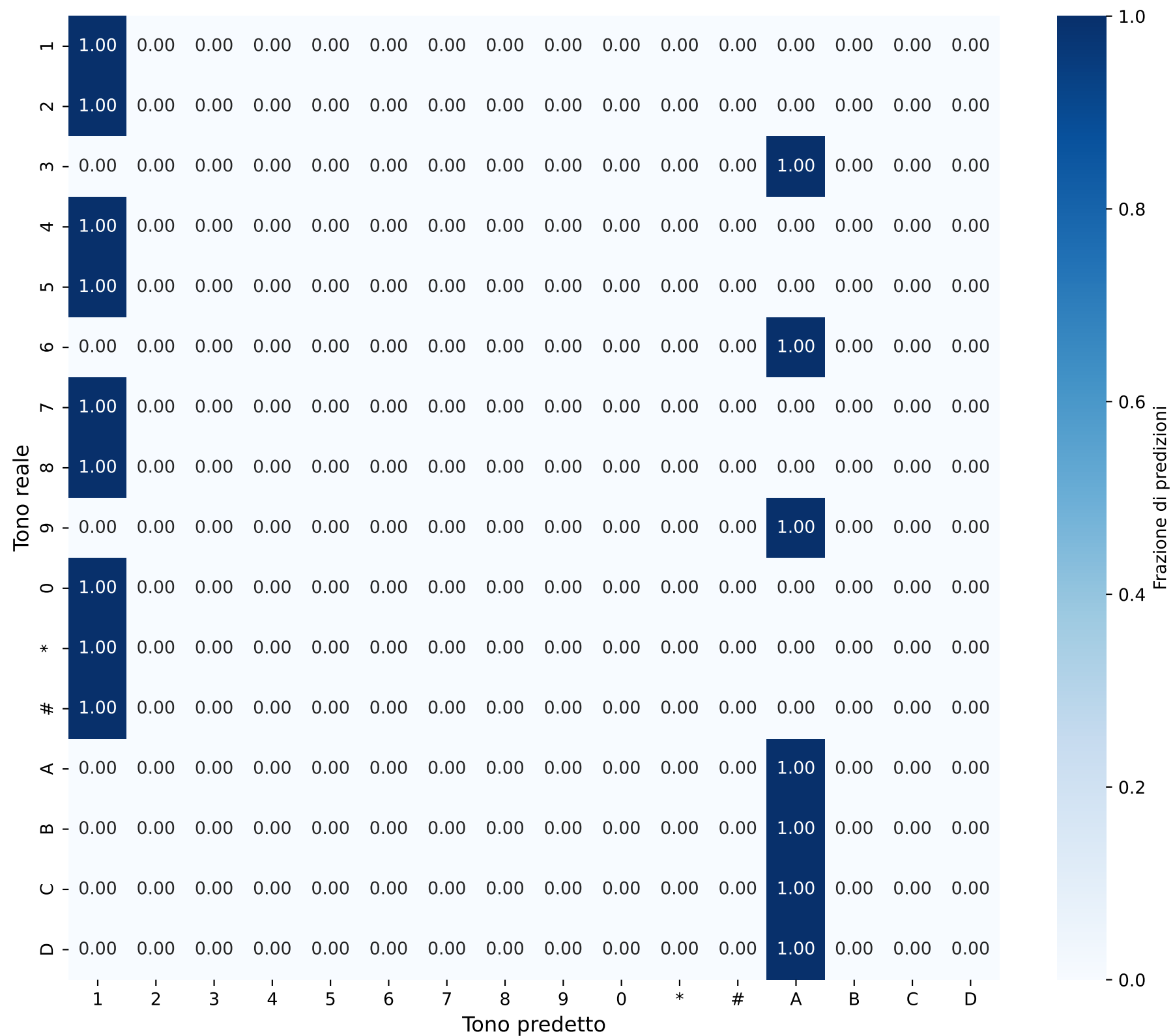
Matrice di Confusione -Singoli Toni Durata: 0.001s
