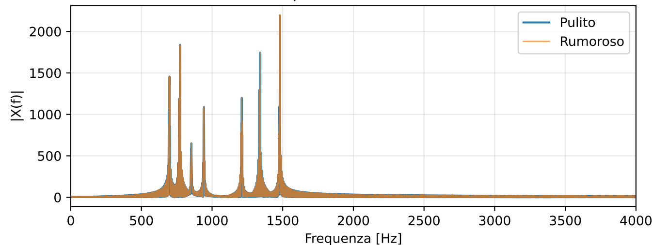
Spettro ( \sigma = 0.2 )
