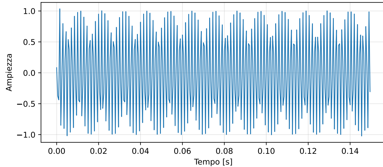
Sottocampionato con filtro anti-alias - F_s = 2000 Hz
