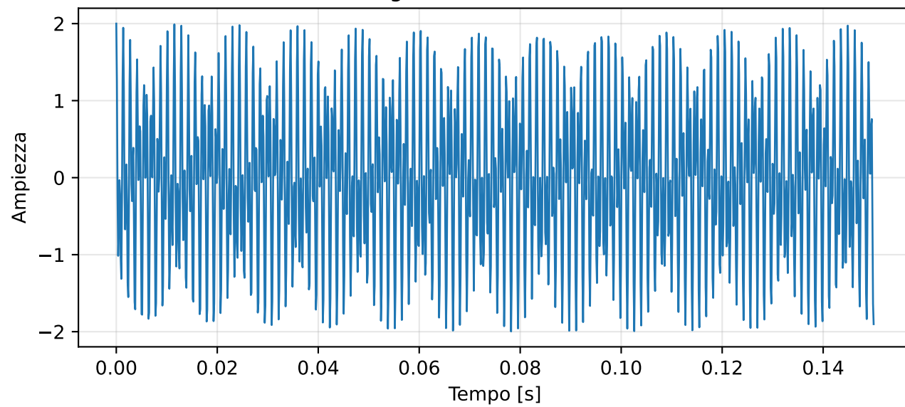
Sottocampionato senza filtro - F_s = 2000 Hz
