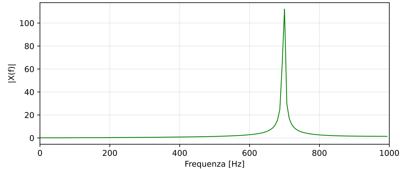
Spettro filtrato - F_s = 2000 Hz
