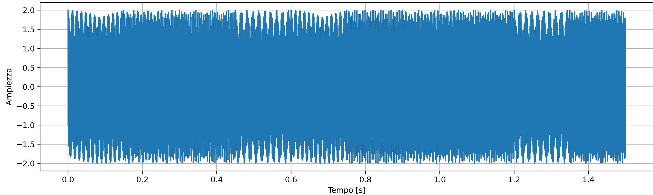
Sequenza DTMF nel dominio del tempo
