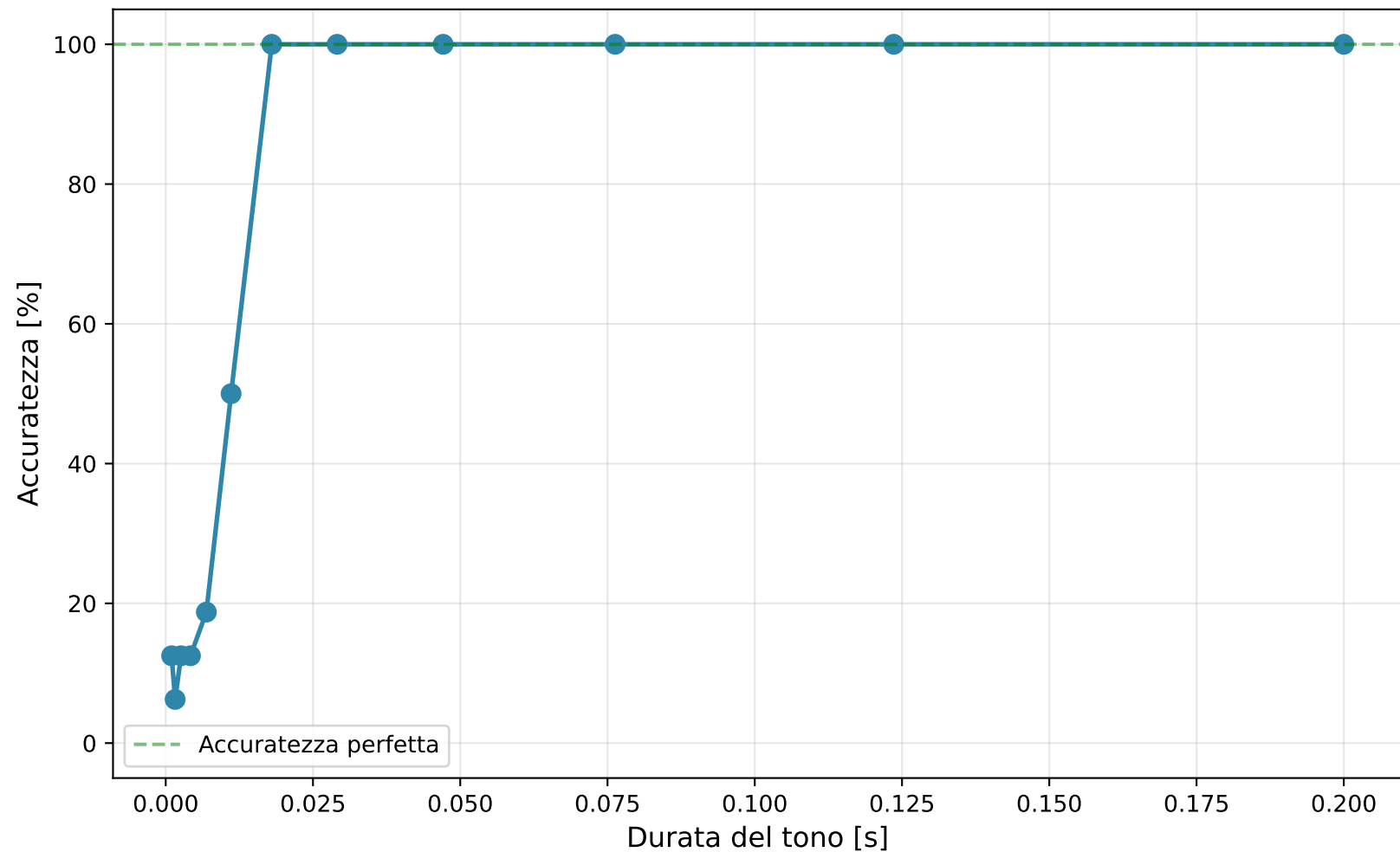
Accuratezza di riconoscimento di singoli toni DTMF al variare della durata
