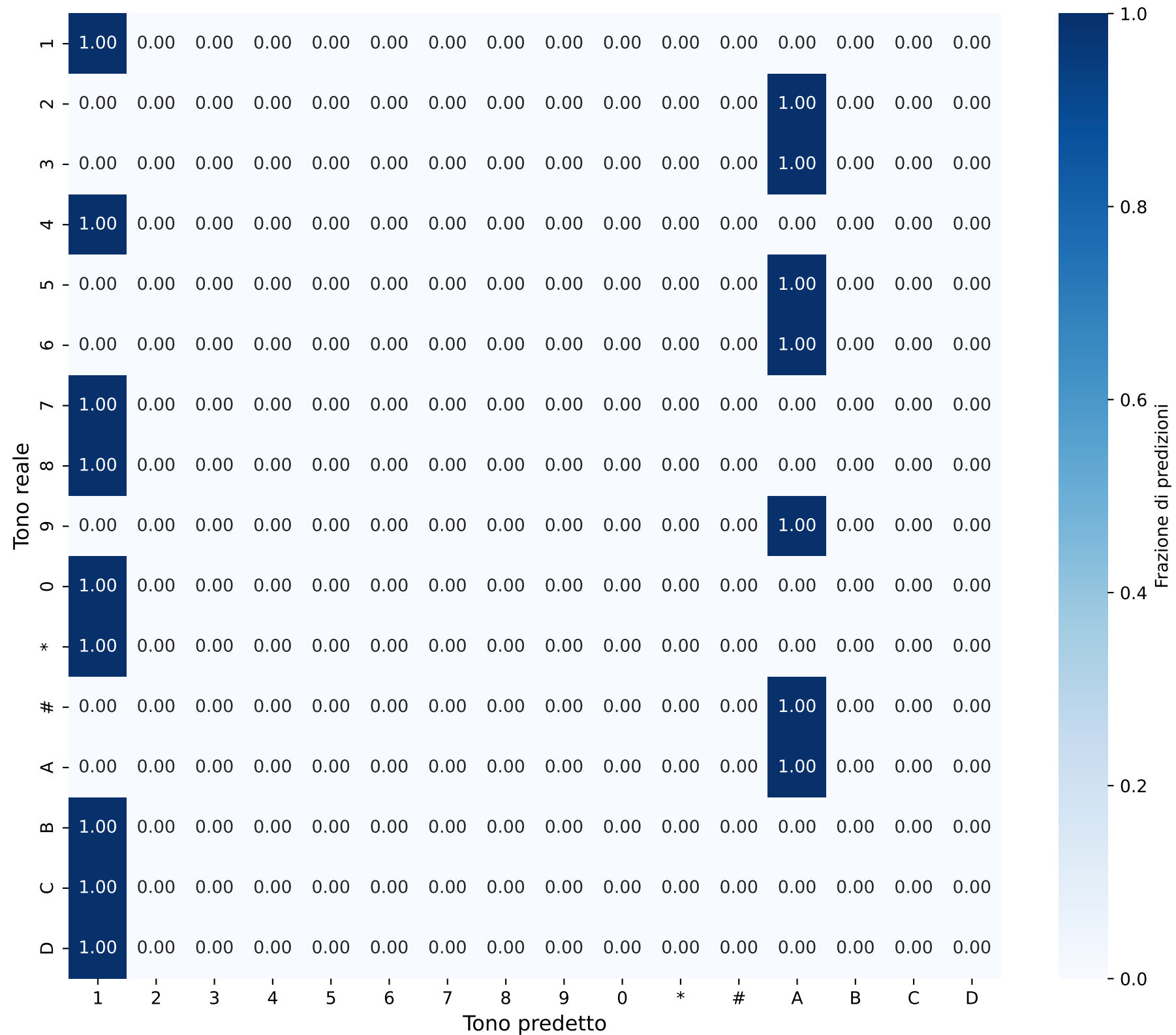
Matrice di Confusione - Sequenze Durata: 0.001114191384195843s
