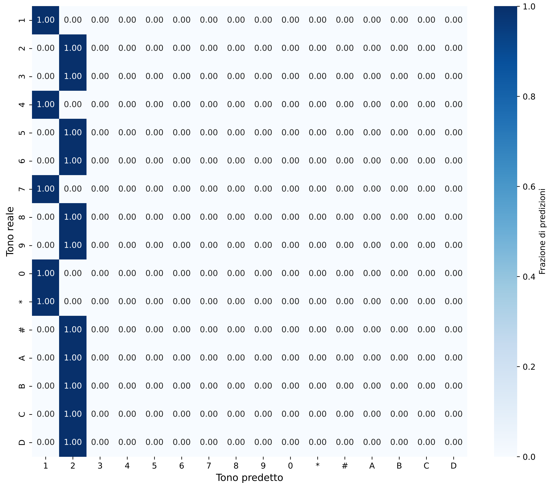
Matrice di Confusione - Sequenze Durata: 0.0017171134070008219s
