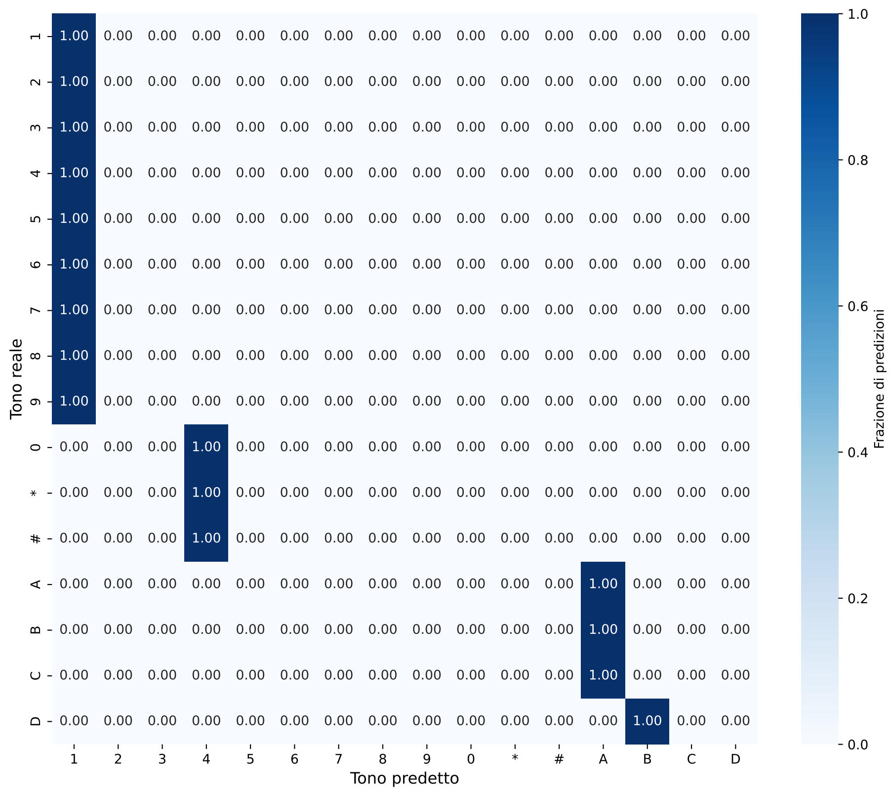
Matrice di Confusione - Sequenze Durata: 0.002646294428699078s
