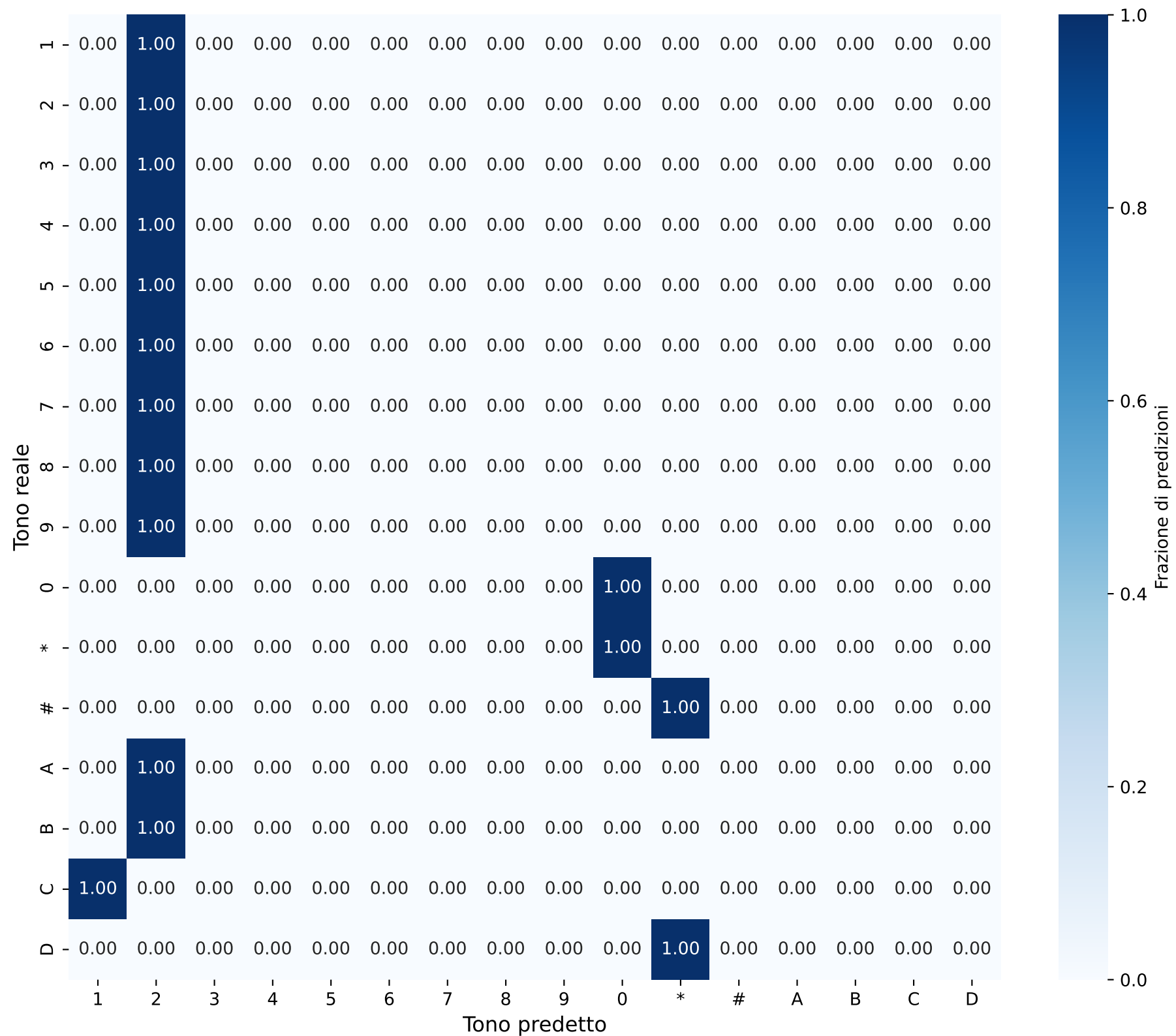
Matrice di Confusione - Sequenze Durata: 0.0027524625874895004s
