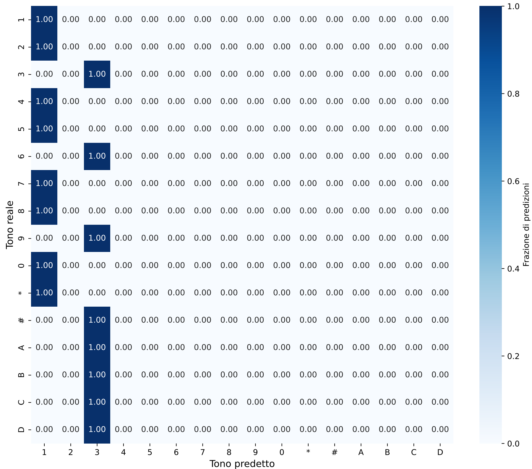
Matrice di Confusione - Sequenze Durata: 0.0029484784525019734s
