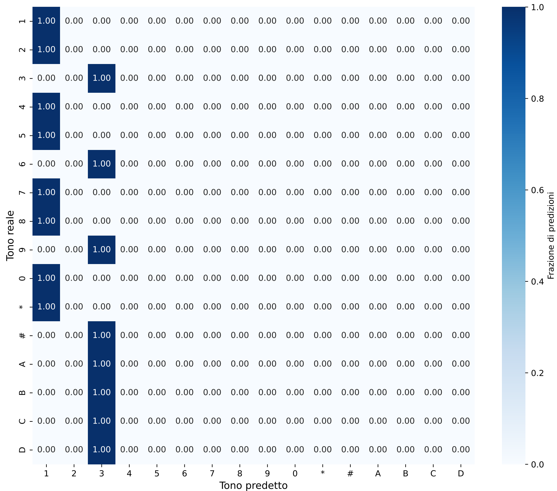
Matrice di Confusione - Sequenze Durata: 0.0029812217553762434s
