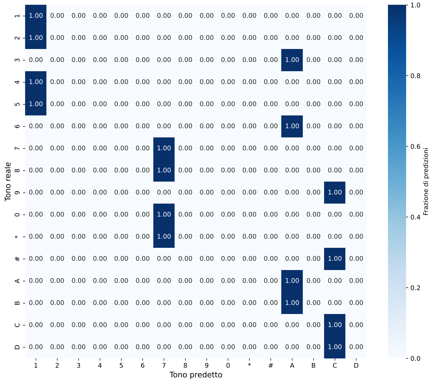
Matrice di Confusione - Sequenze Durata: 0.003019040530780201s
