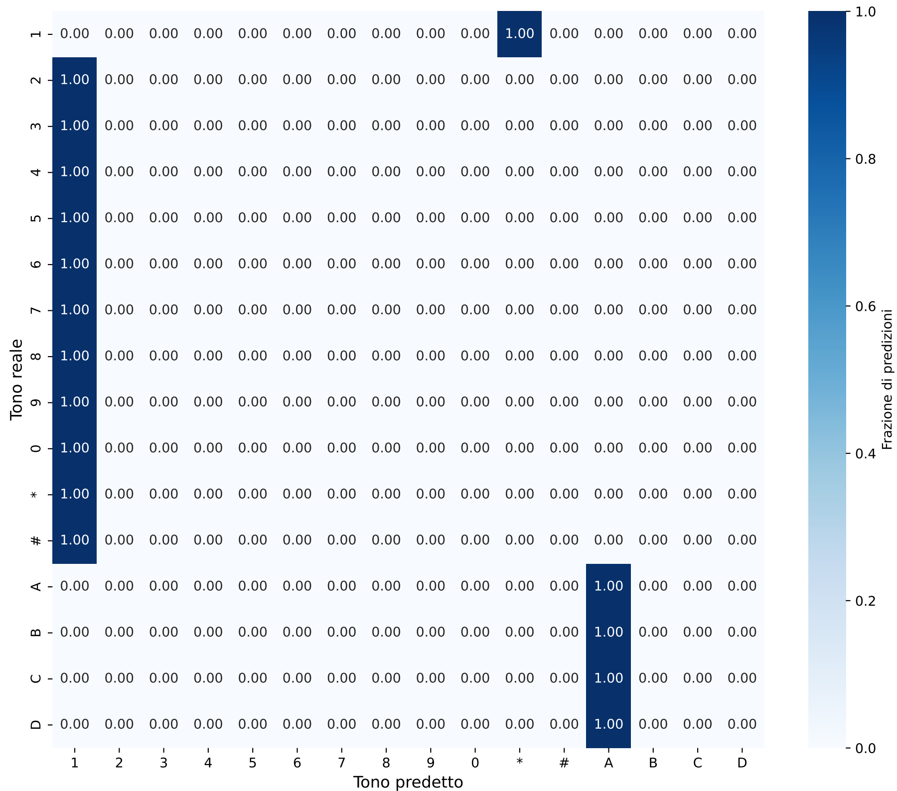
Matrice di Confusione - Sequenze Durata: 0.003419951893353393s
