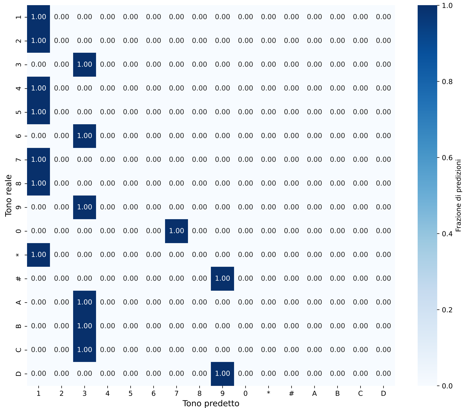
Matrice di Confusione - Sequenze Durata: 0.0037092697468885587s
