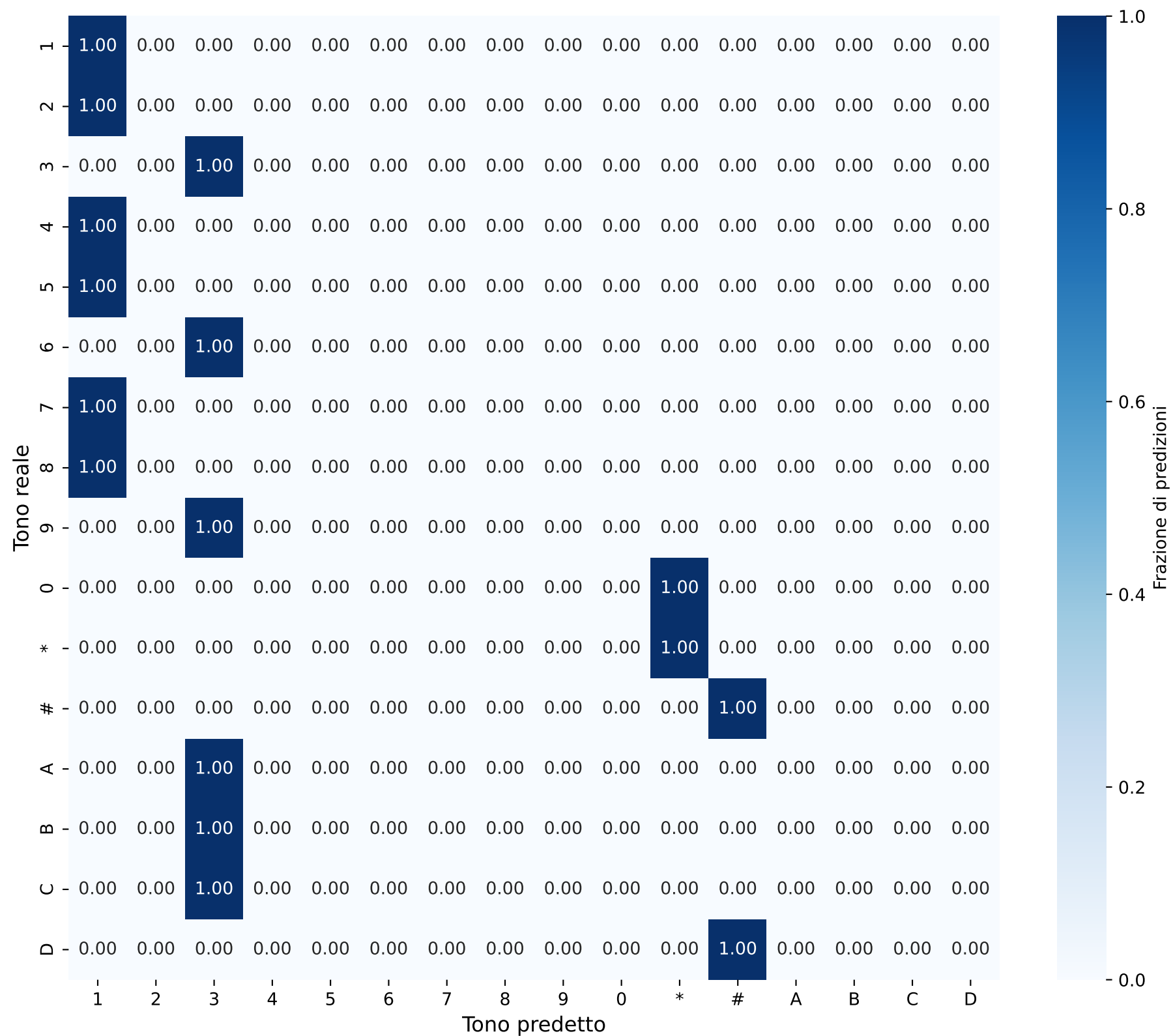
Matrice di Confusione - Sequenze Durata: 0.0037880251477647015s
