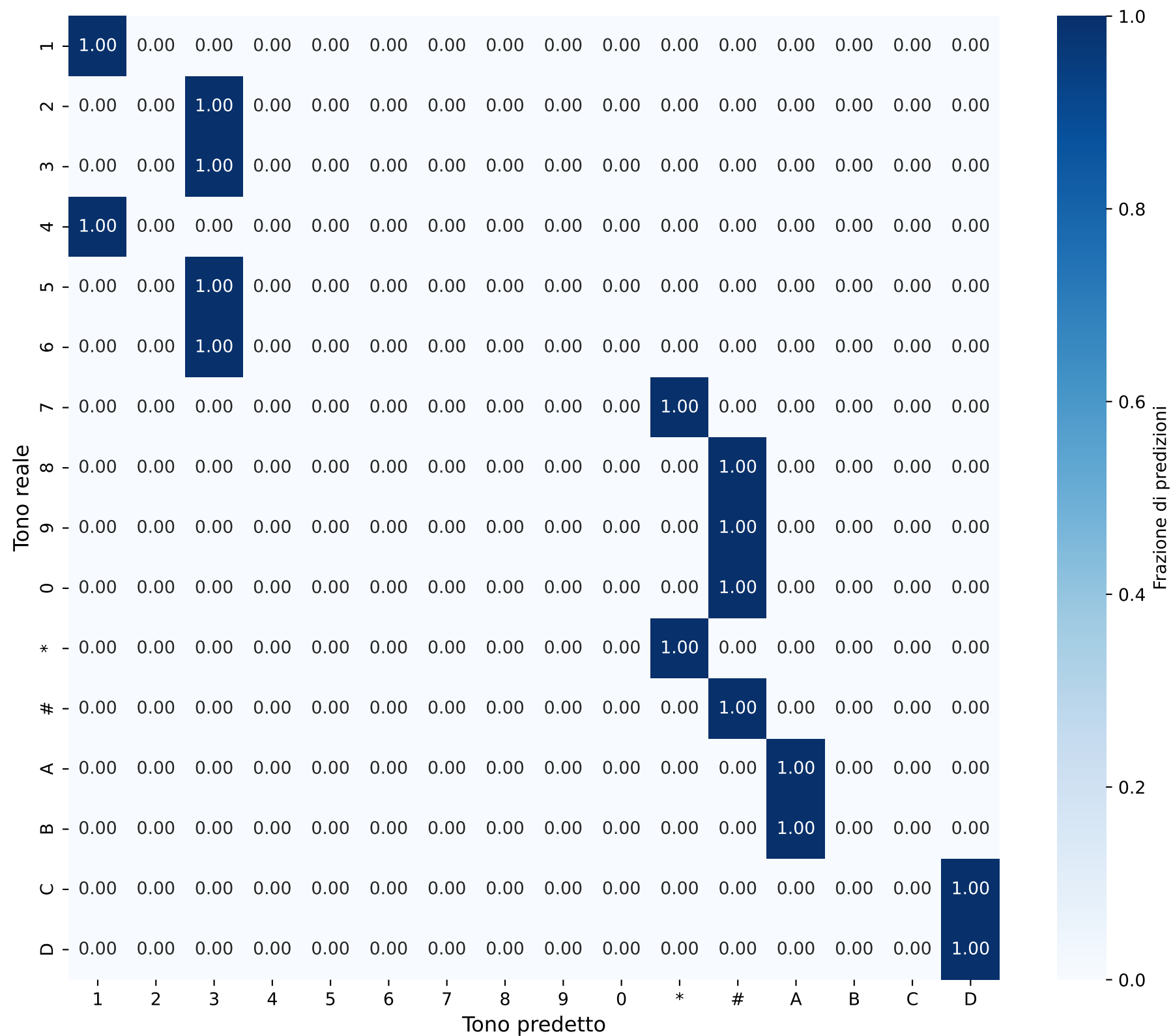
Matrice di Confusione - Sequenze Durata: 0.004102850673341442s
