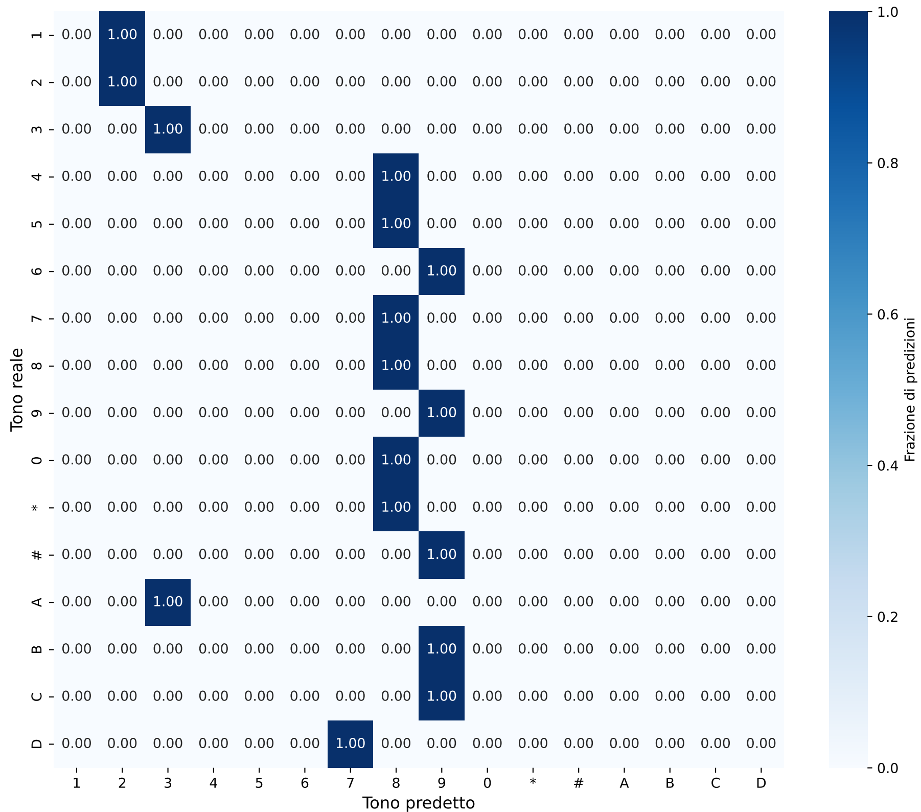
Matrice di Confusione - Sequenze Durata: 0.004543987642390772s
