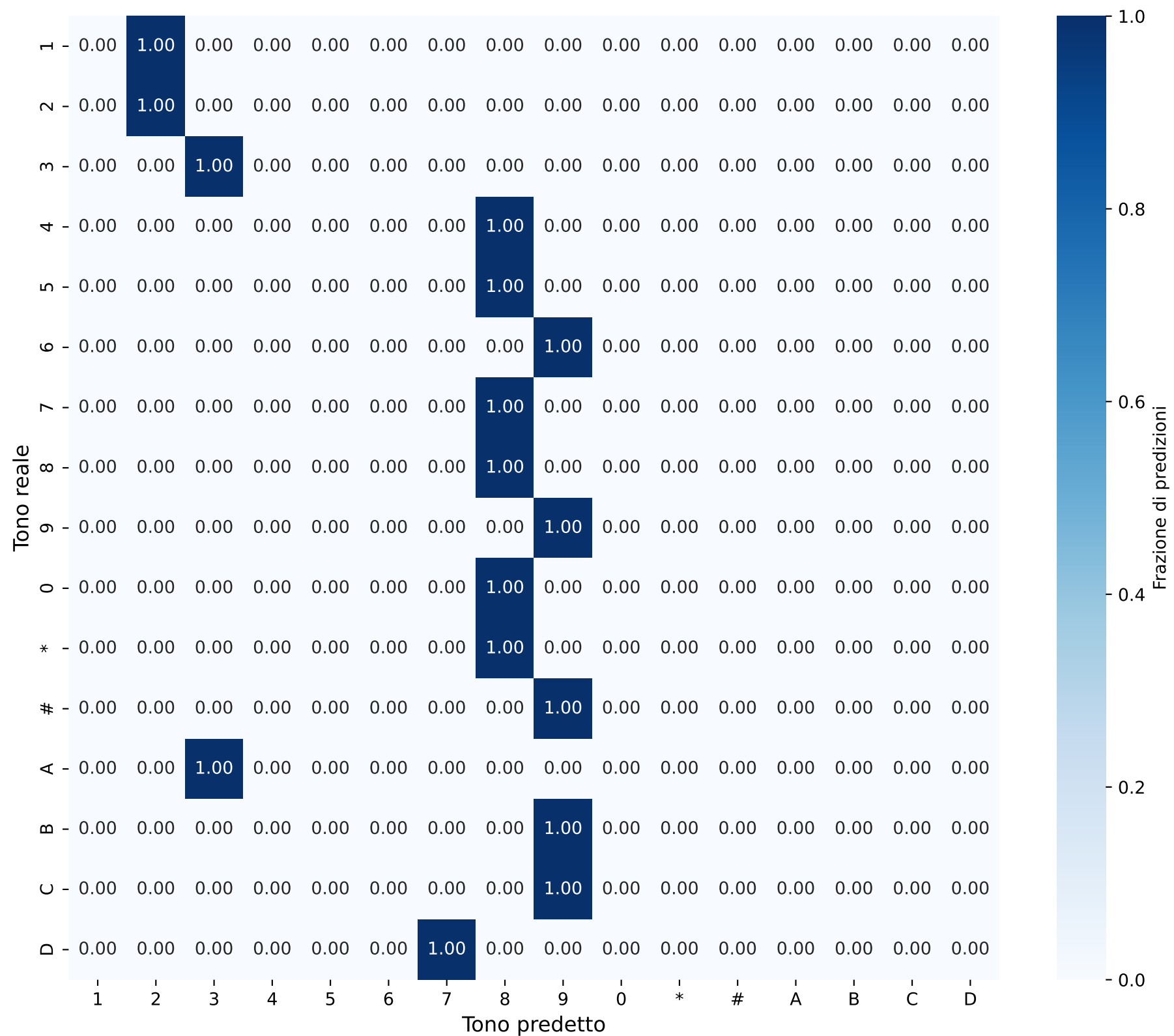
Matrice di Confusione - Sequenze Durata: 0.004557302863246793s
