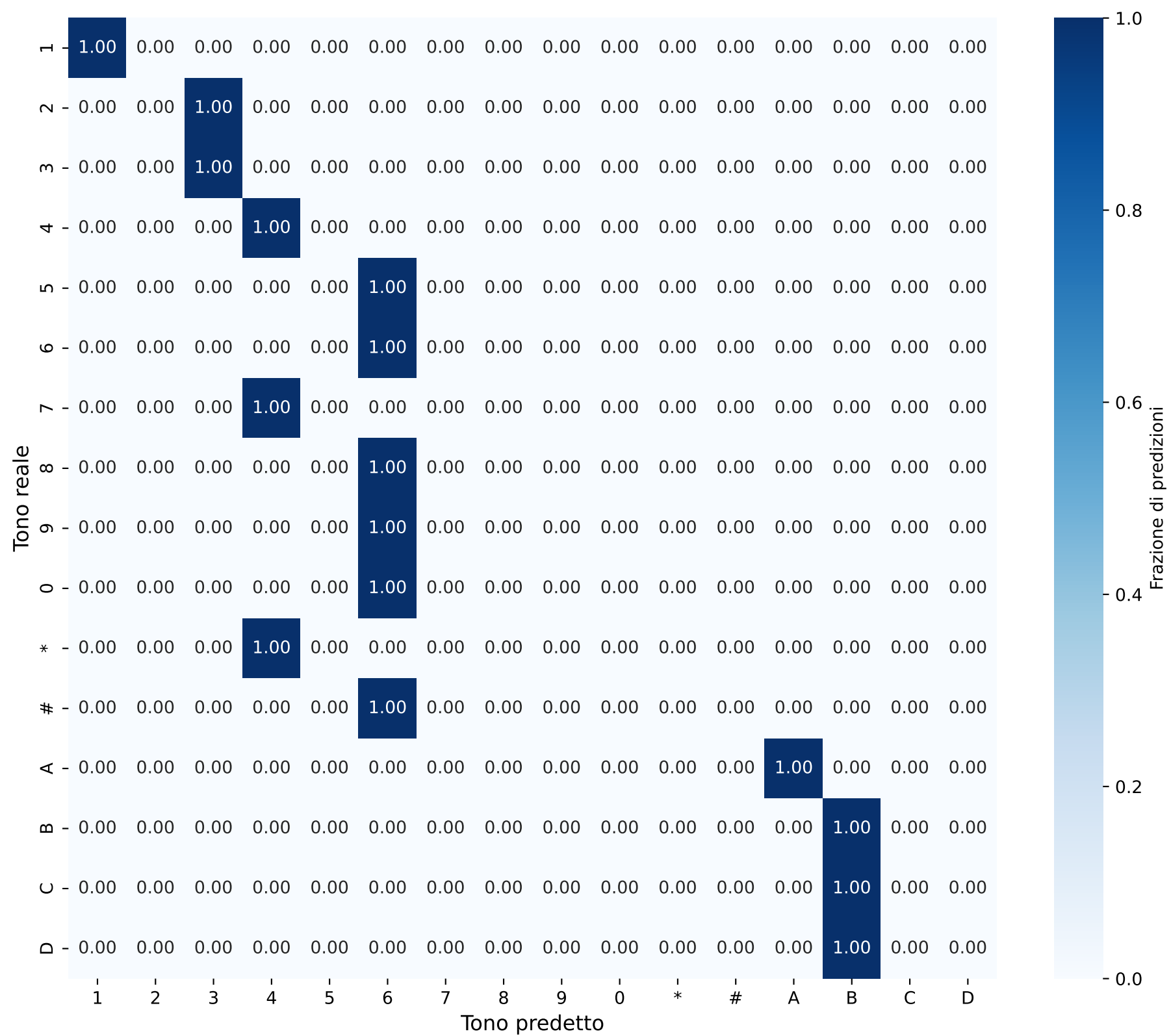
Matrice di Confusione - Sequenze Durata: 0.004813172483469571s
