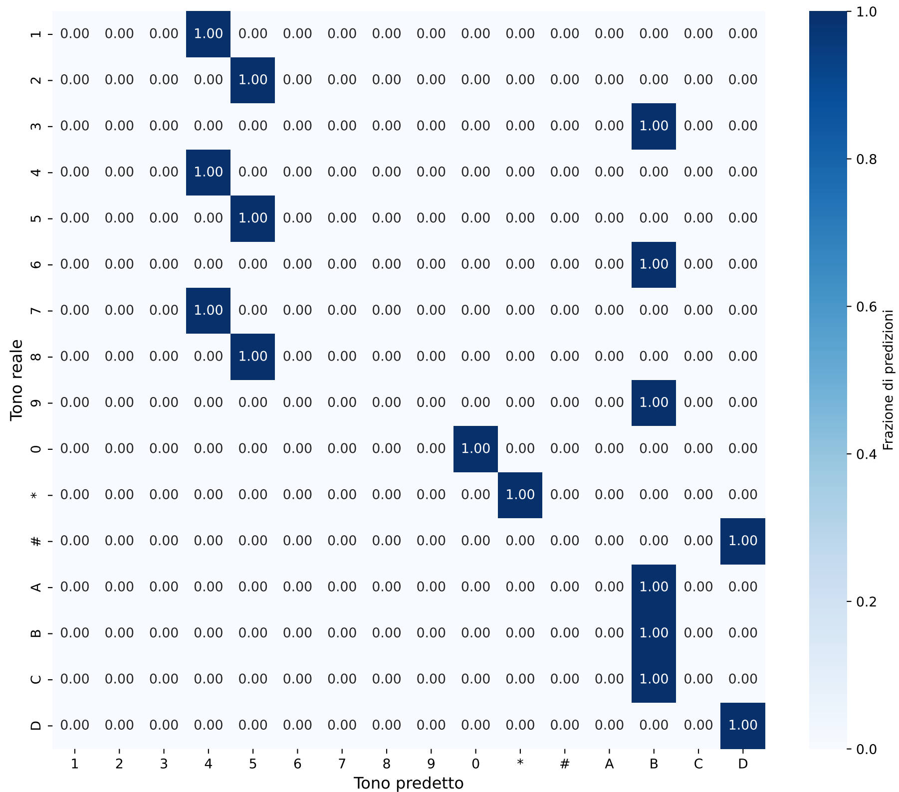
Matrice di Confusione - Sequenze Durata: 0.005062871881044174s
