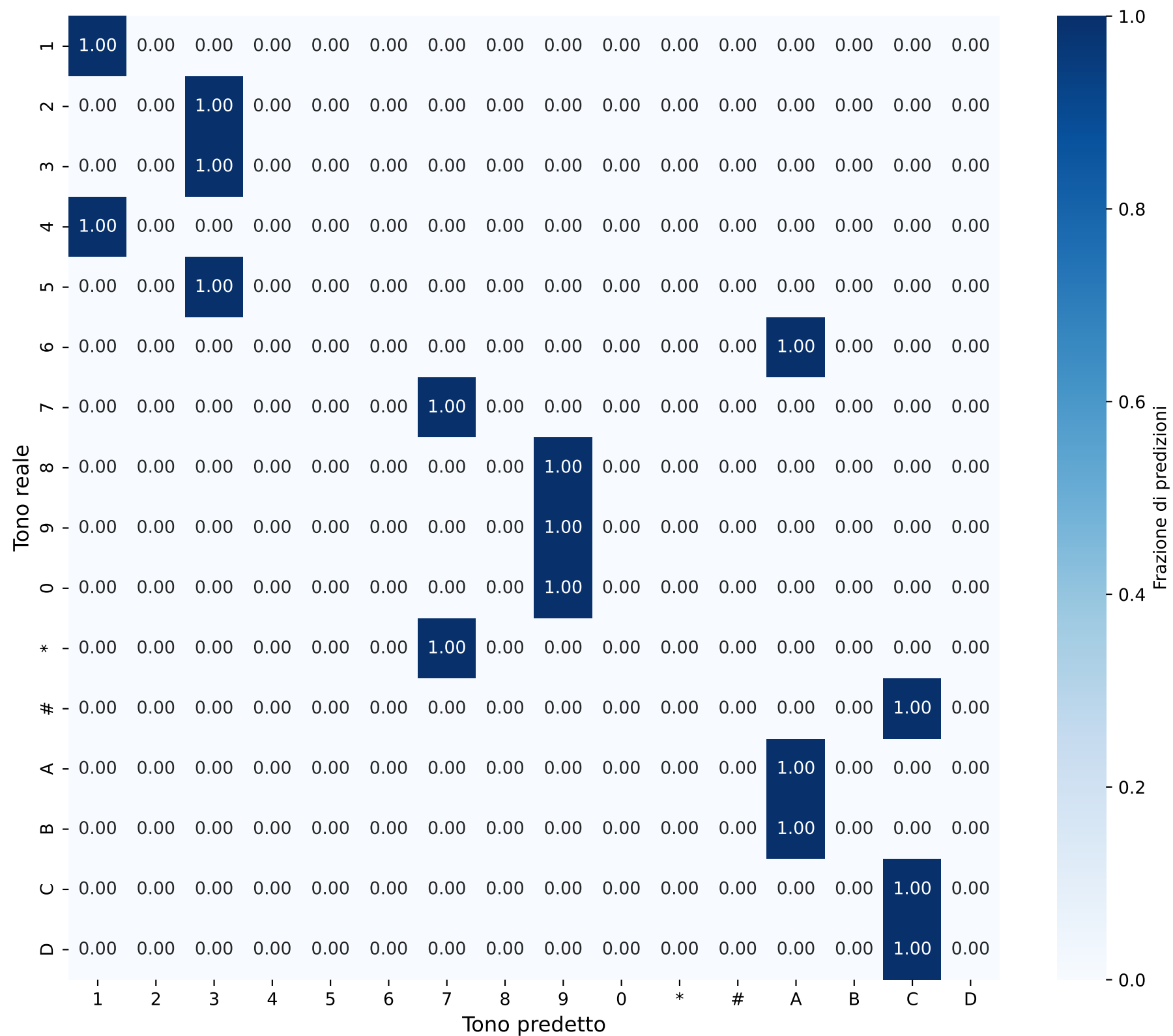
Matrice di Confusione - Sequenze Durata: 0.005599217852726687s
