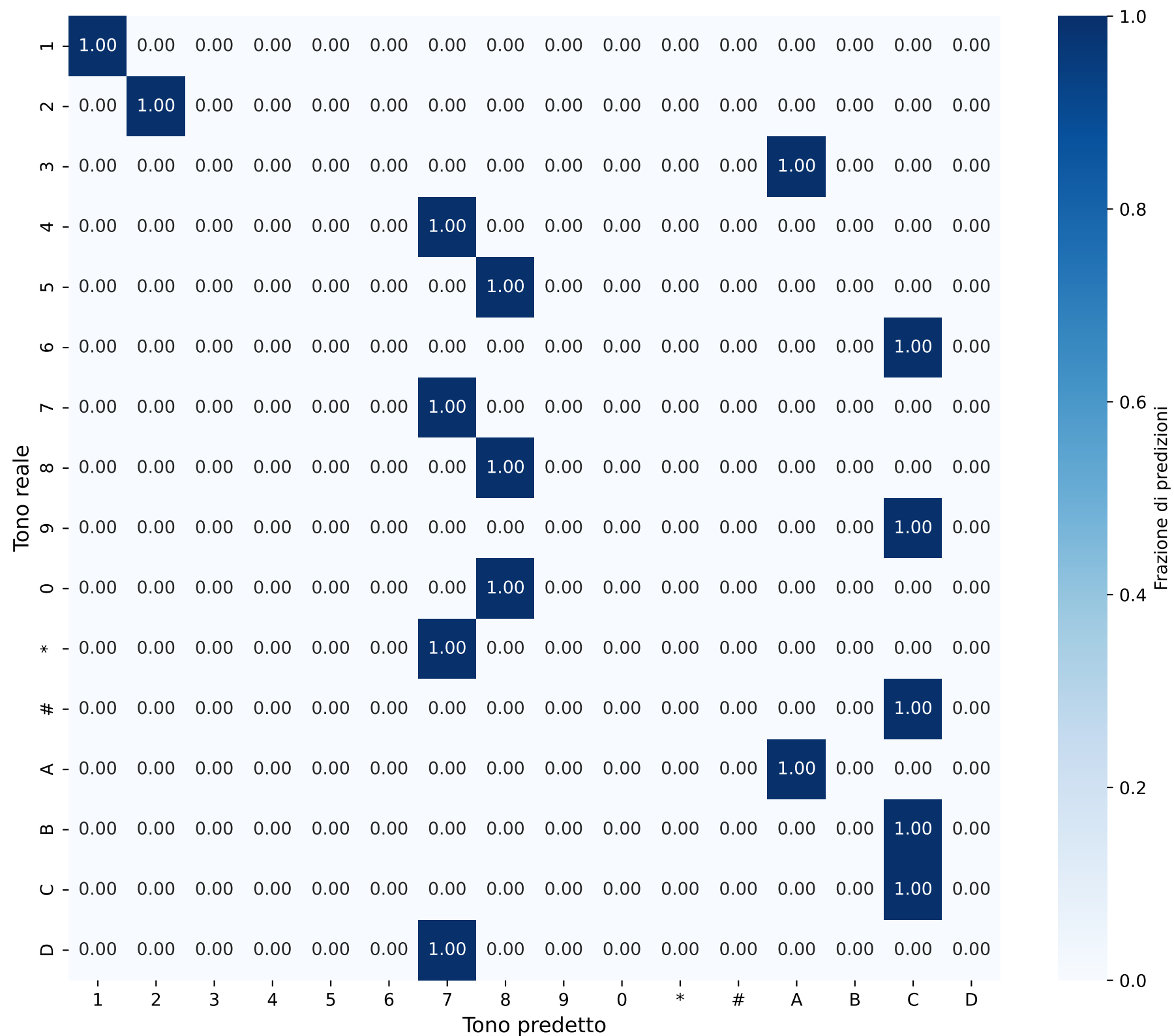
Matrice di Confusione - Sequenze Durata: 0.005848035476425728s
