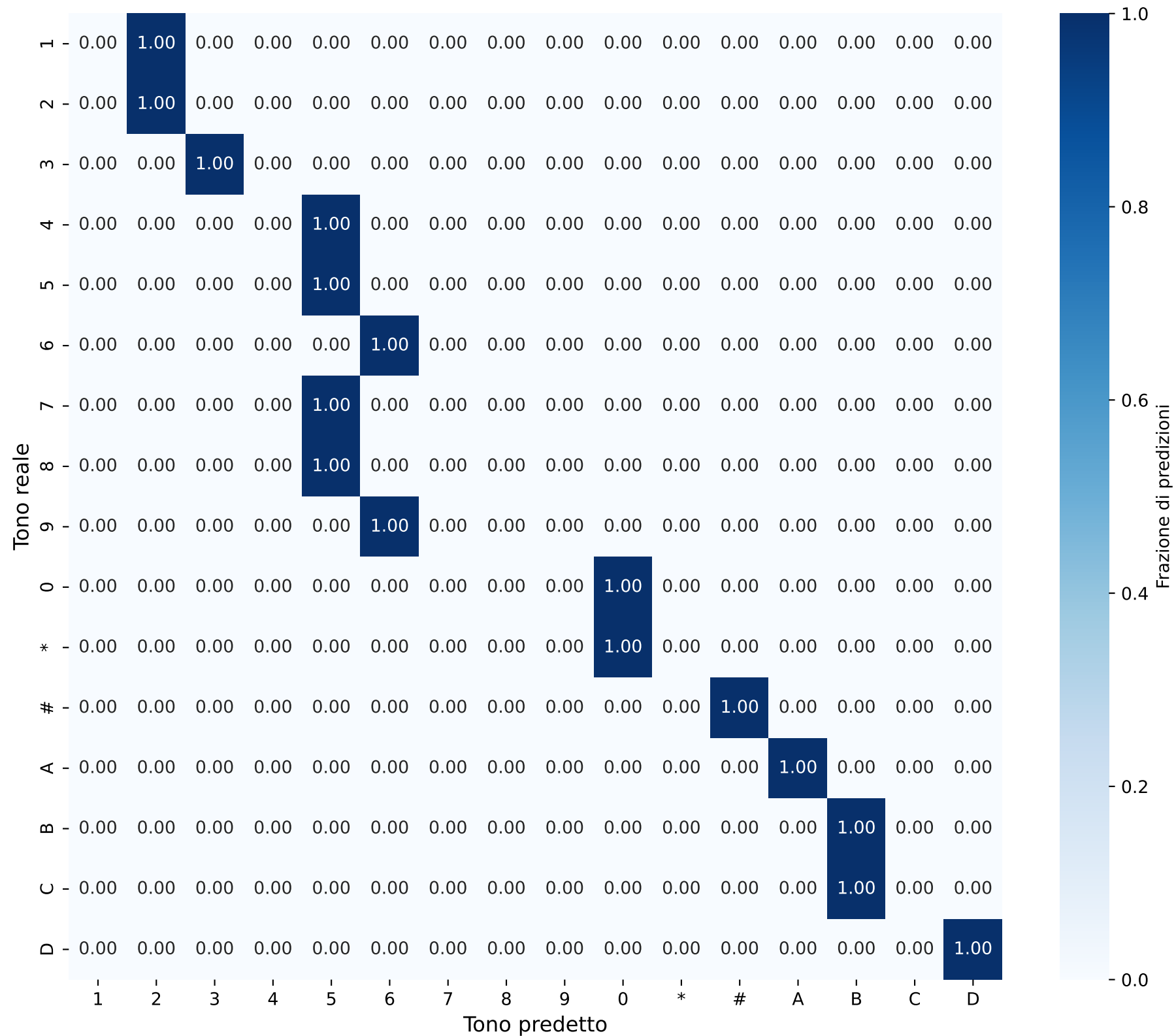
Matrice di Confusione - Sequenze Durata: 0.0061157538432127885s
