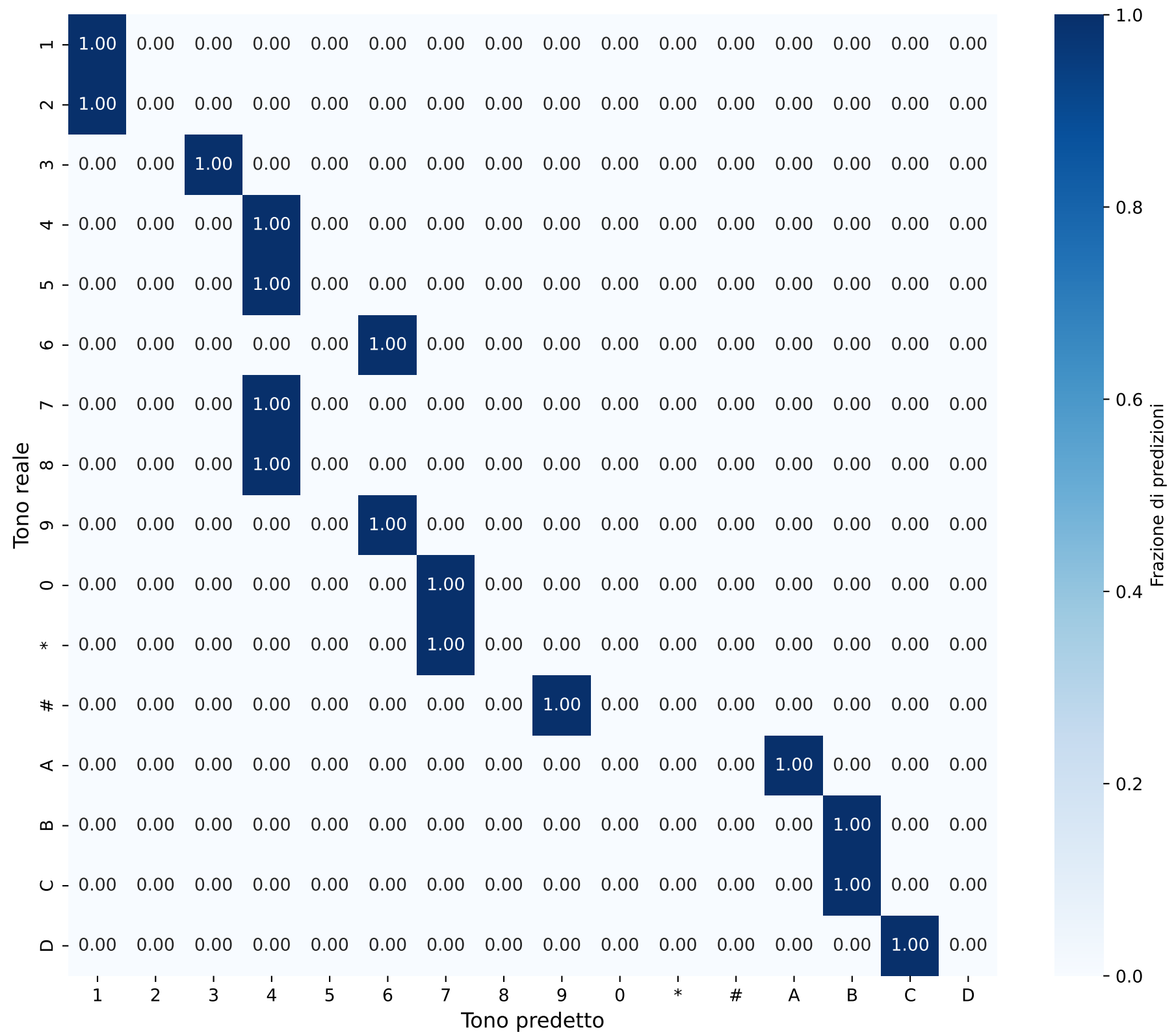
Matrice di Confusione - Sequenze Durata: 0.008416691823869163s
