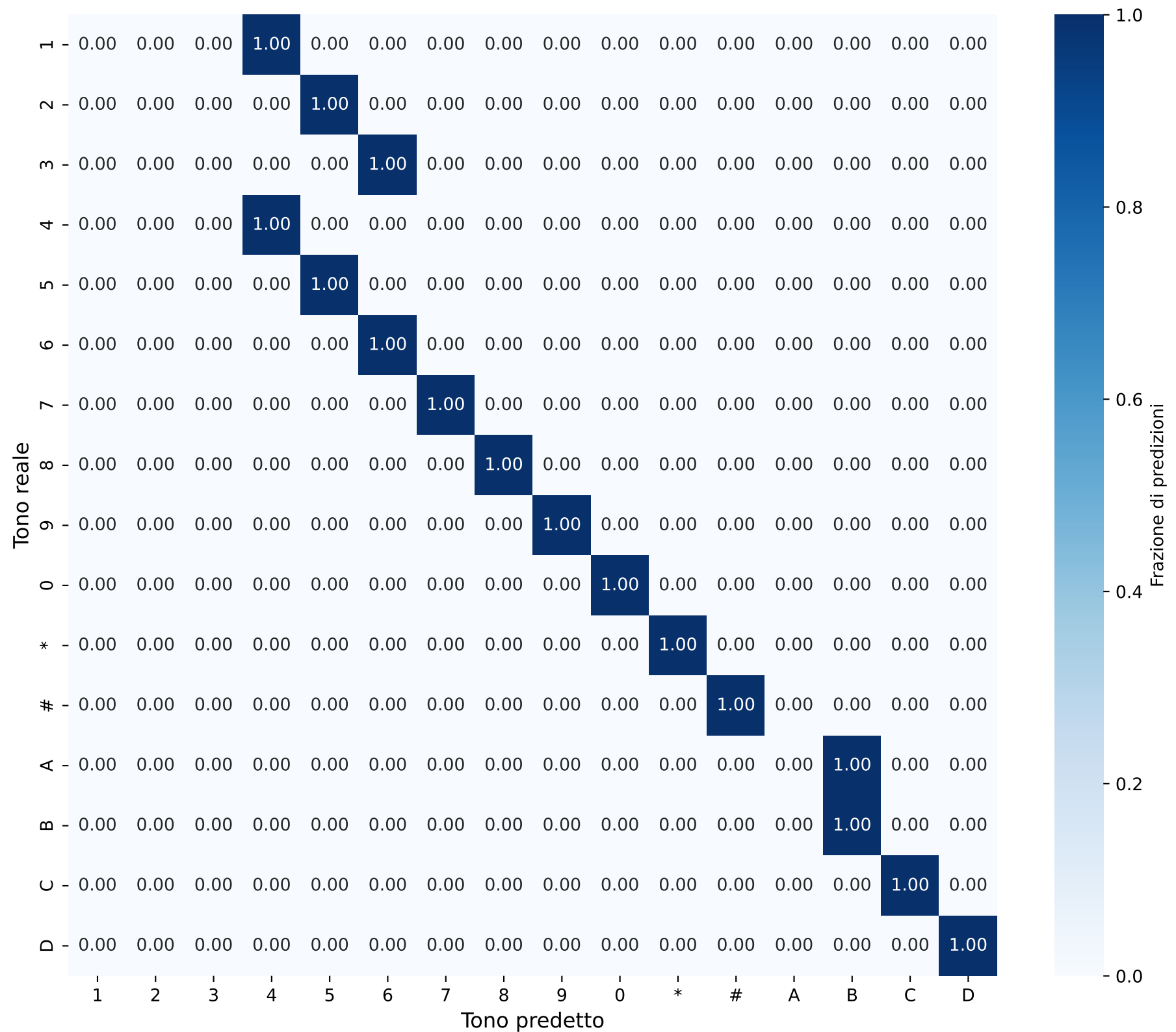
Matrice di Confusione - Sequenze Durata: 0.01079233725255818s
