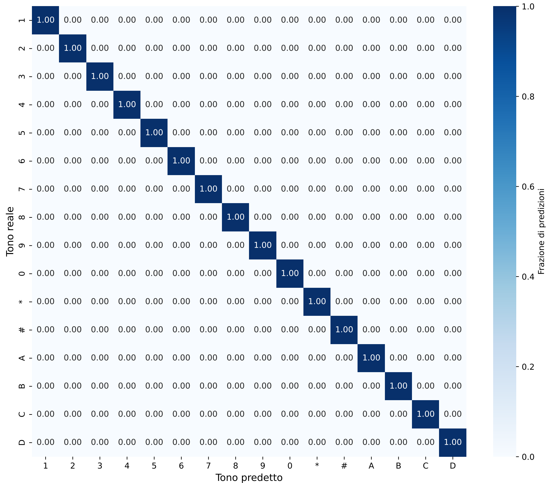
Matrice di Confusione - Sequenze Durata: 0.012024729182136158s
