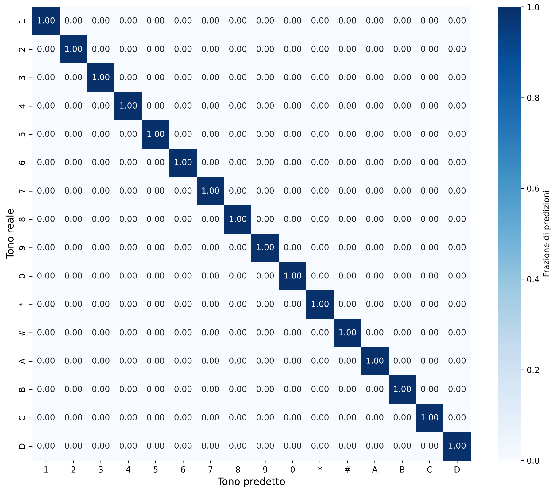
Matrice di Confusione - Sequenze Durata: 0.012599210498948734s
