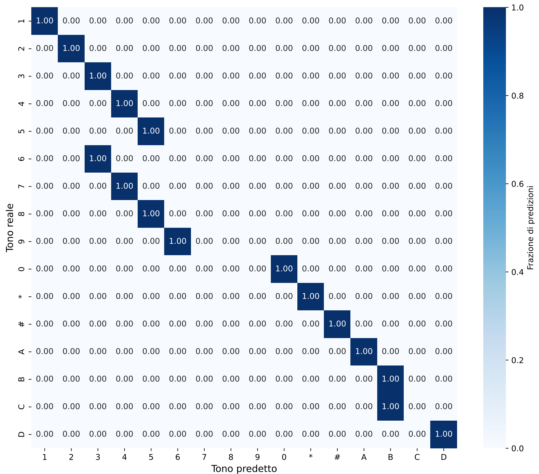
Matrice di Confusione - Sequenze Durata: 0.01567562028114663s
