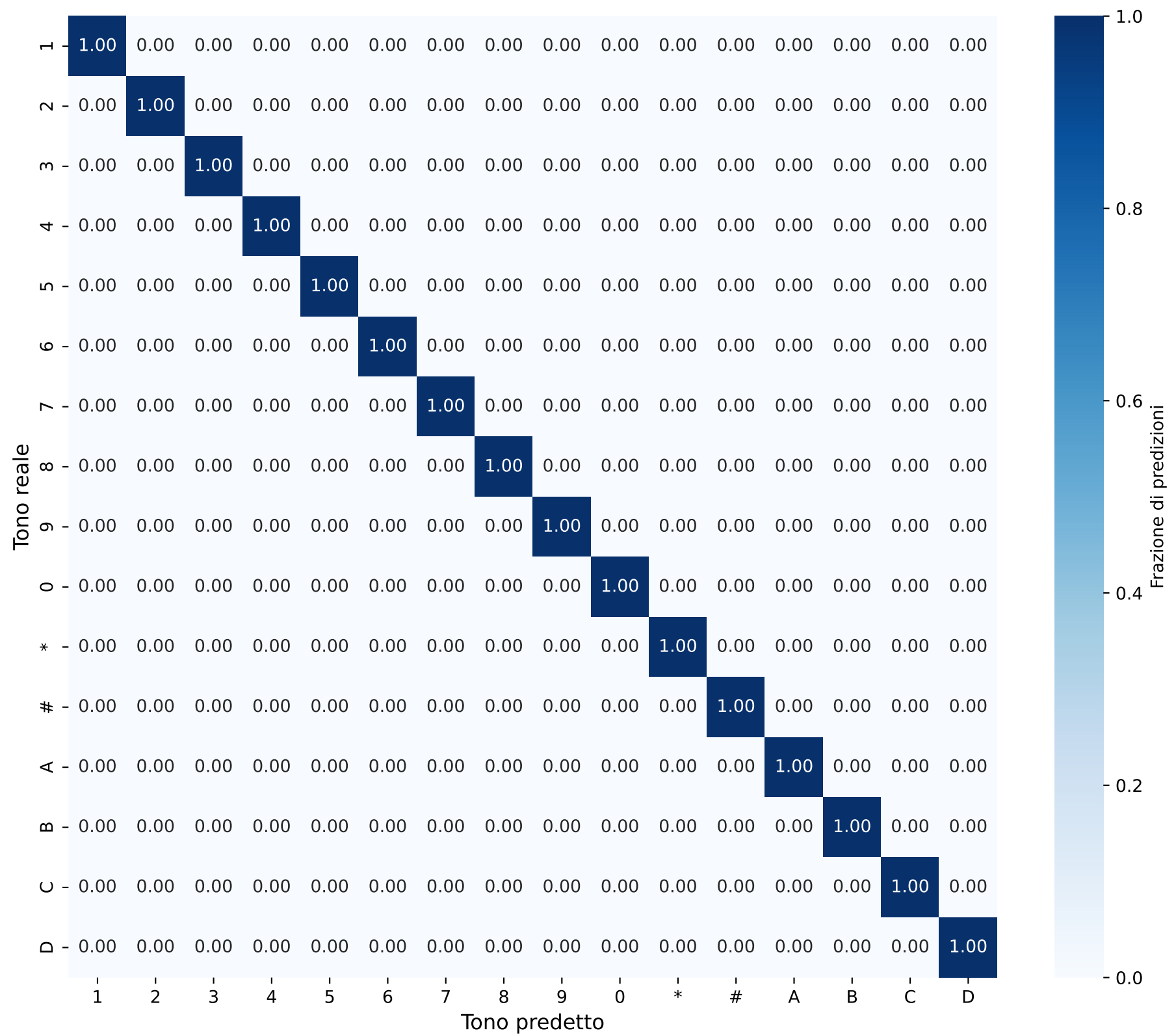
Matrice di Confusione - Sequenze Durata: 0.017266214858434503s
