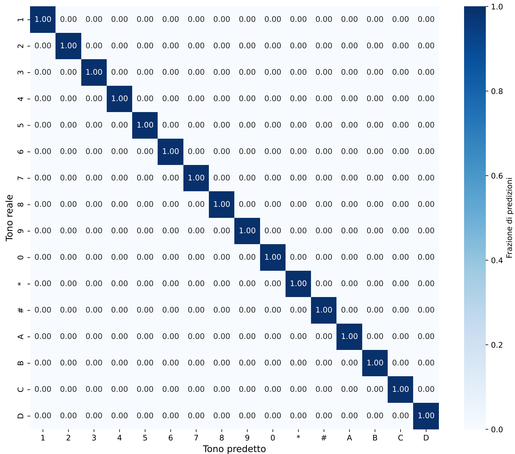
Matrice di Confusione - Sequenze Durata: 0.027144176165949066s
