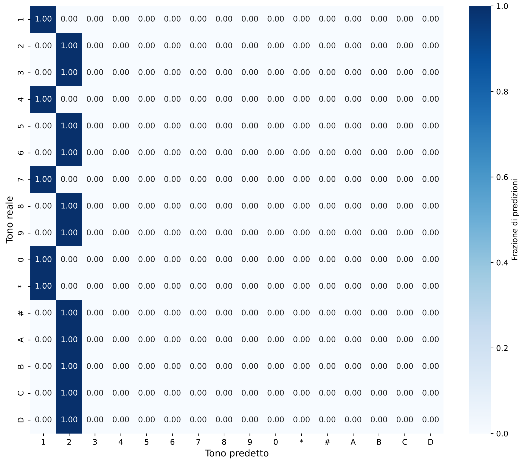
Matrice di Confusione - Singoli Toni Durata: 0.0017171134070008219s
