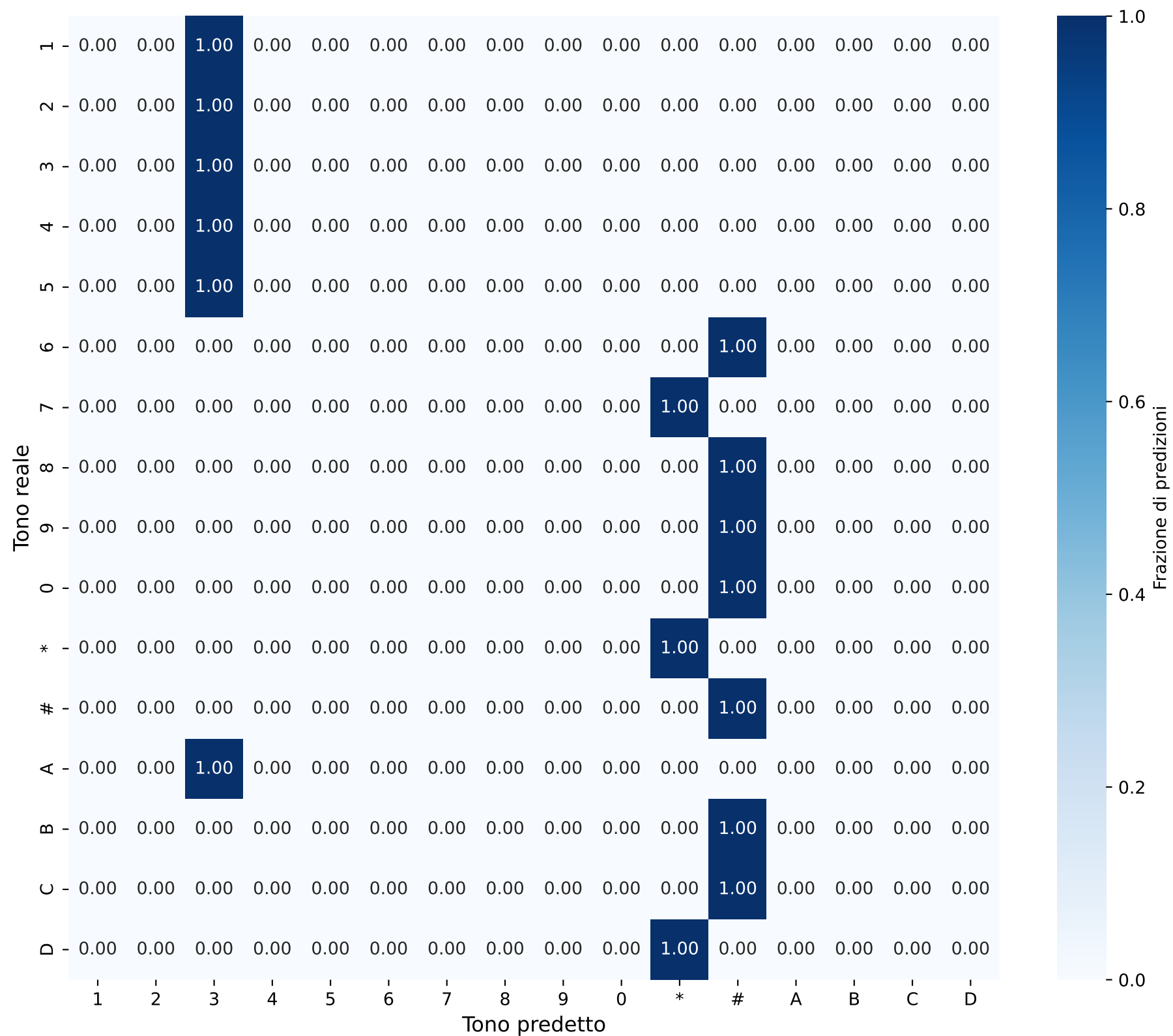
Matrice di Confusione - Singoli Toni Durata: 0.001801648230654412s
