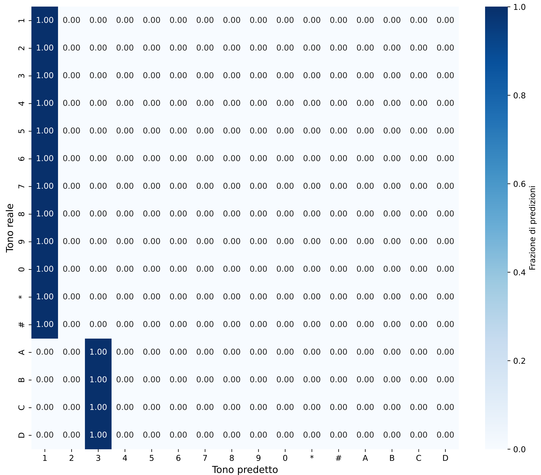
Matrice di Confusione - Singoli Toni Durata: 0.002166221454872082s
